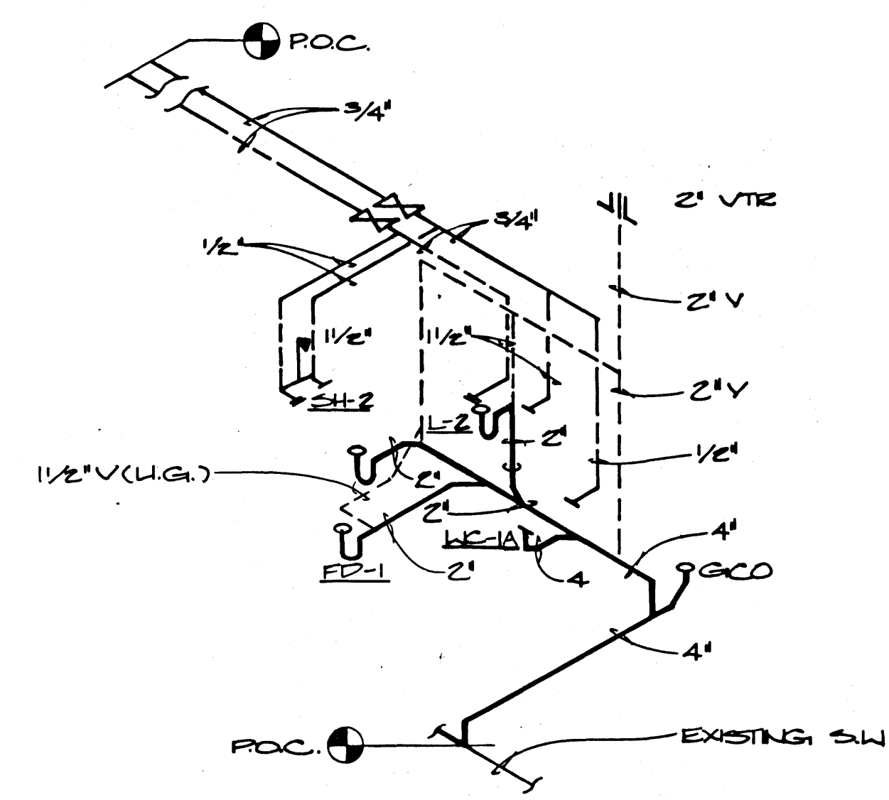
PIPING DIAGRAM N.T.S.
