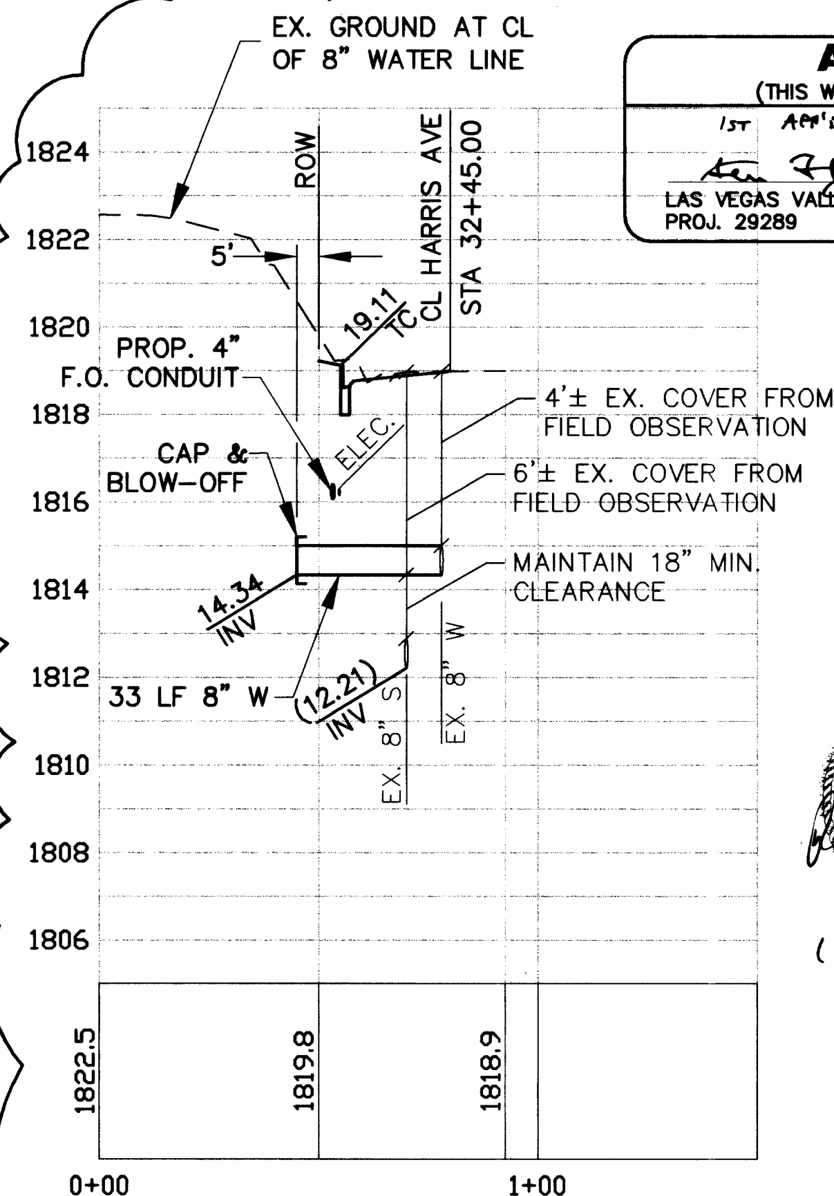
F Water Lateral Profile - Harris Ave Scale: Horiz. 1" = 30' Scale: Vert. 1" = 3'
