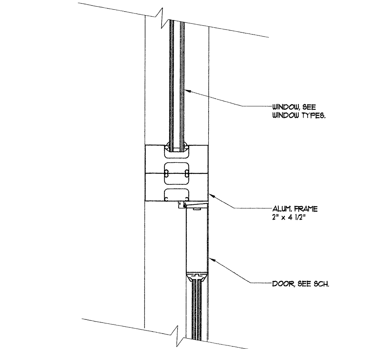
11 Head - Jamb Sim. Scale: 3/4"=1'-0" 08400-02 AT-011
