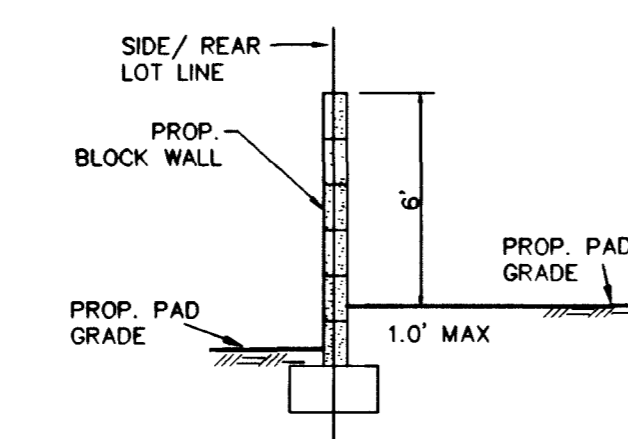
2 BLOCK WALL SECTION DETAIL (N.T.S.)
