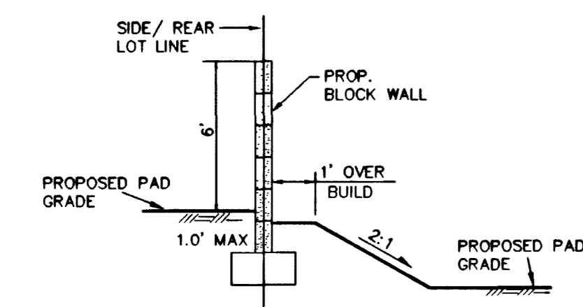
1 BLOCK WALL SECTION DETAIL (N.T.S.)
