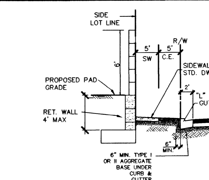
4 RETAINING WALL SECTION DETAIL (N.T.S.)
