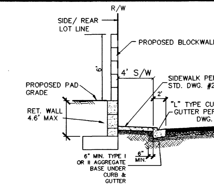
3 RETAINING WALL SECTION DETAIL (N.T.S.)
