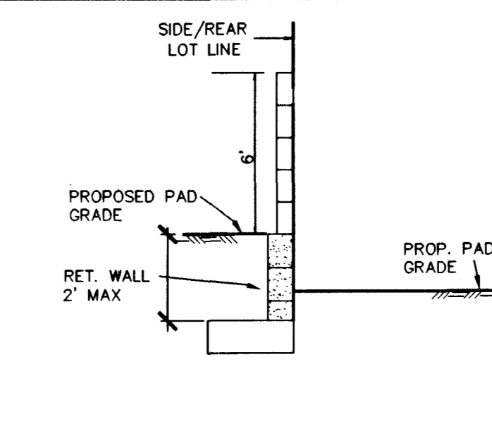
5 RETAINING WALL SECTION DETAIL (N.T.S.)
