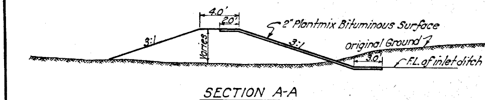
PAVED DIKE
