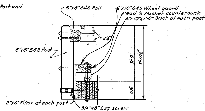
SECTION D-D
