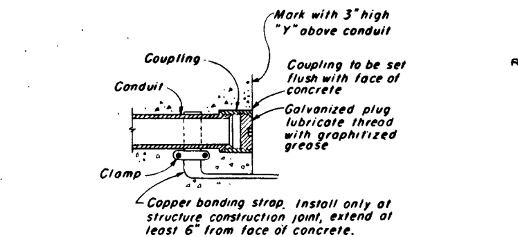
DETAIL "B" CONDUIT TERMINATION
