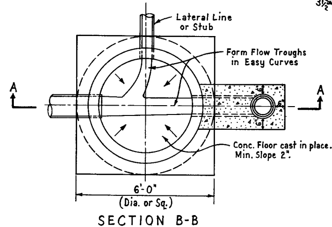
TYPE 3 MANHOLE
