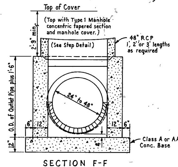
TYPE 4 MANHOLE
