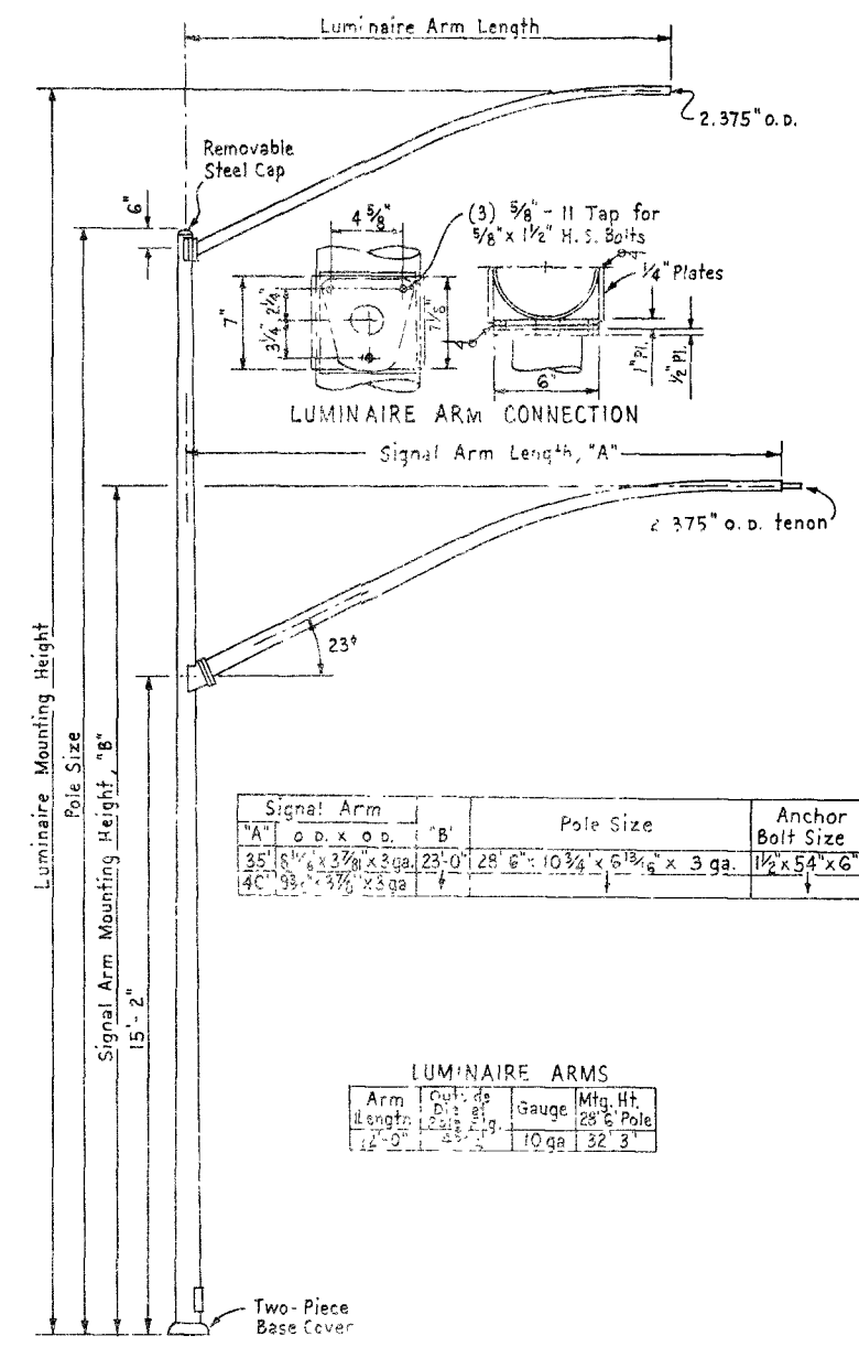
POLE TYPE 24
