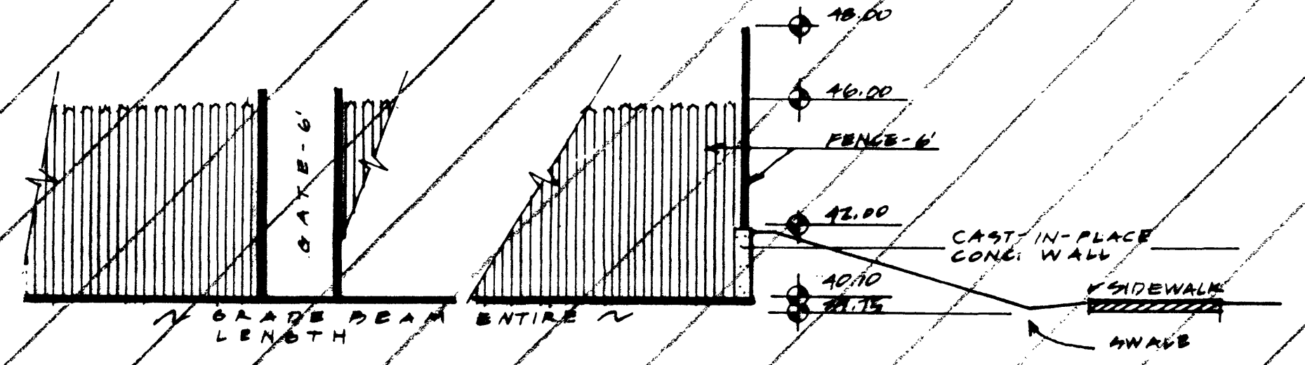
SECTION @ SNACK BAR - SECTION A-A VERT.: 1/4"=1'-0" HORIZ.: 1/8"=1'-0"
