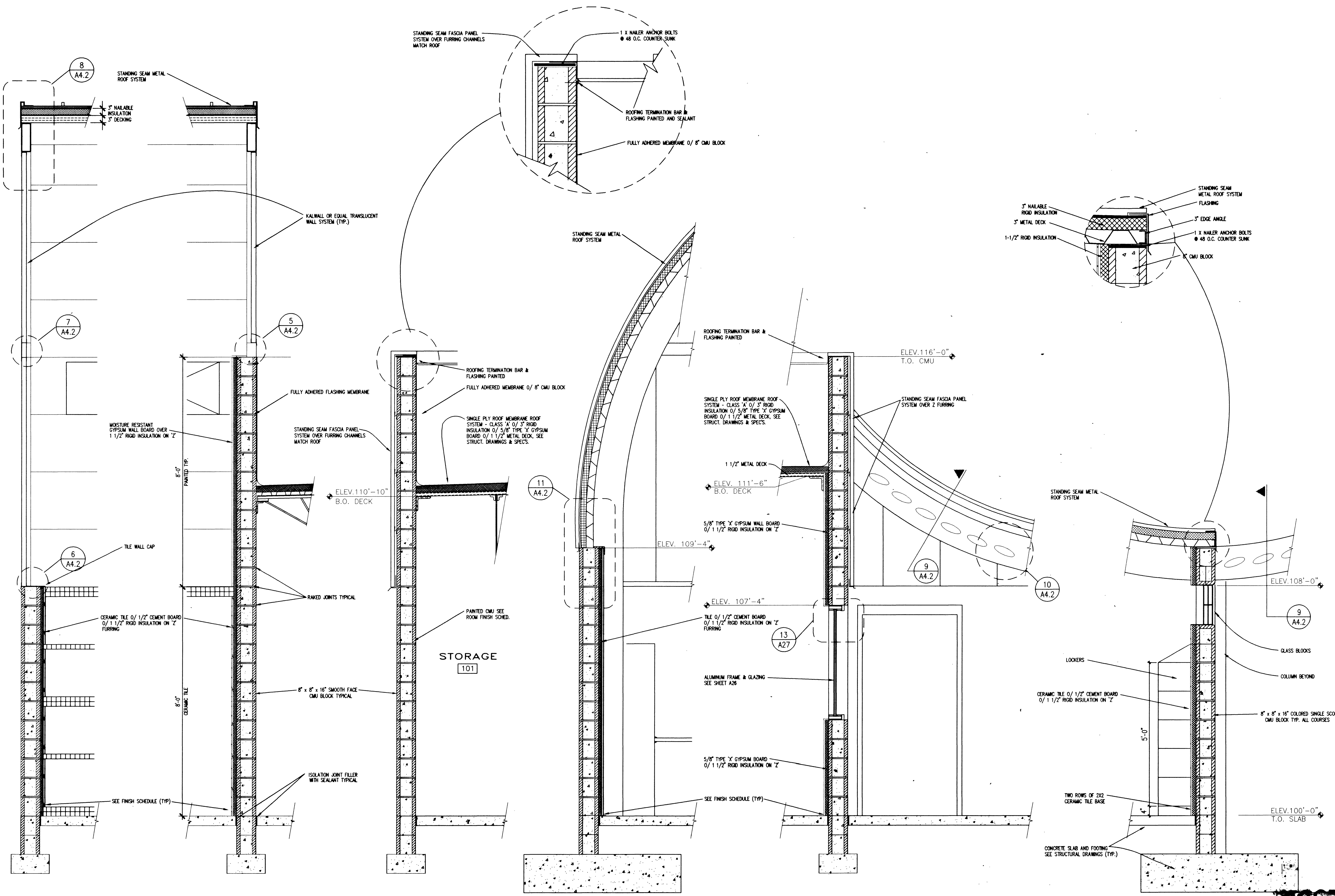
1 WALL SECTION A4.1 SCALE: 3/4" = 1'-0"
