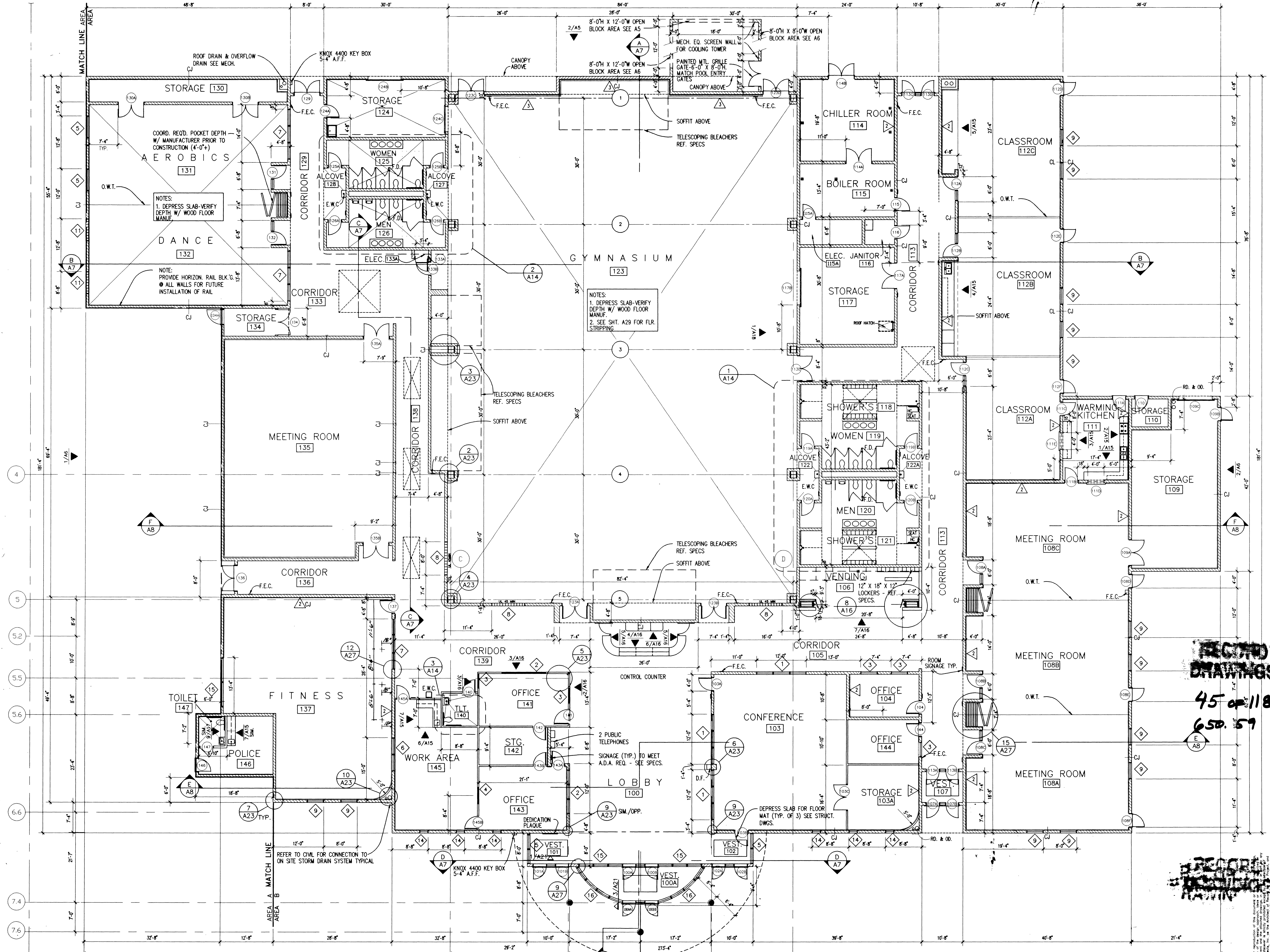
1 FLOOR PLAN AREA B A3 SCALE: 1/8" = 1'-0"
