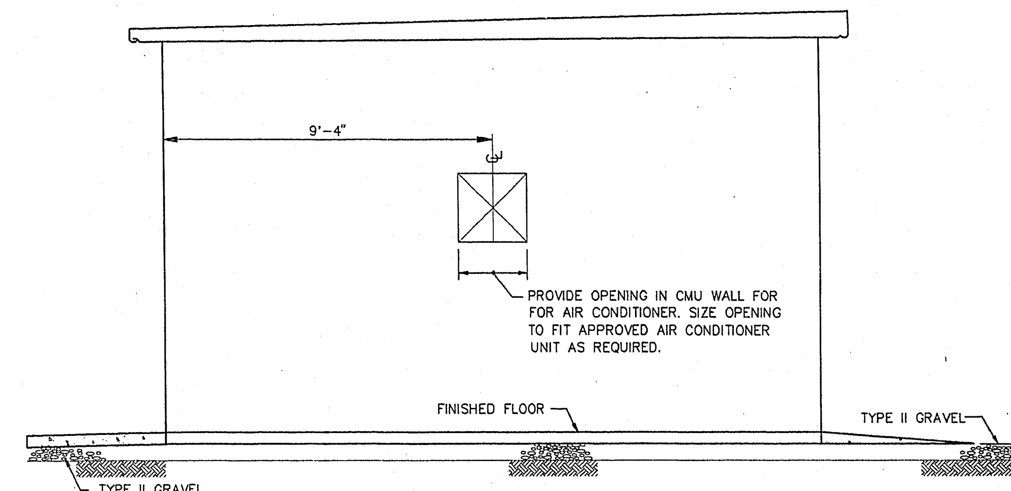
ELEVATION SCALE: 3/8" = 1'-0"
