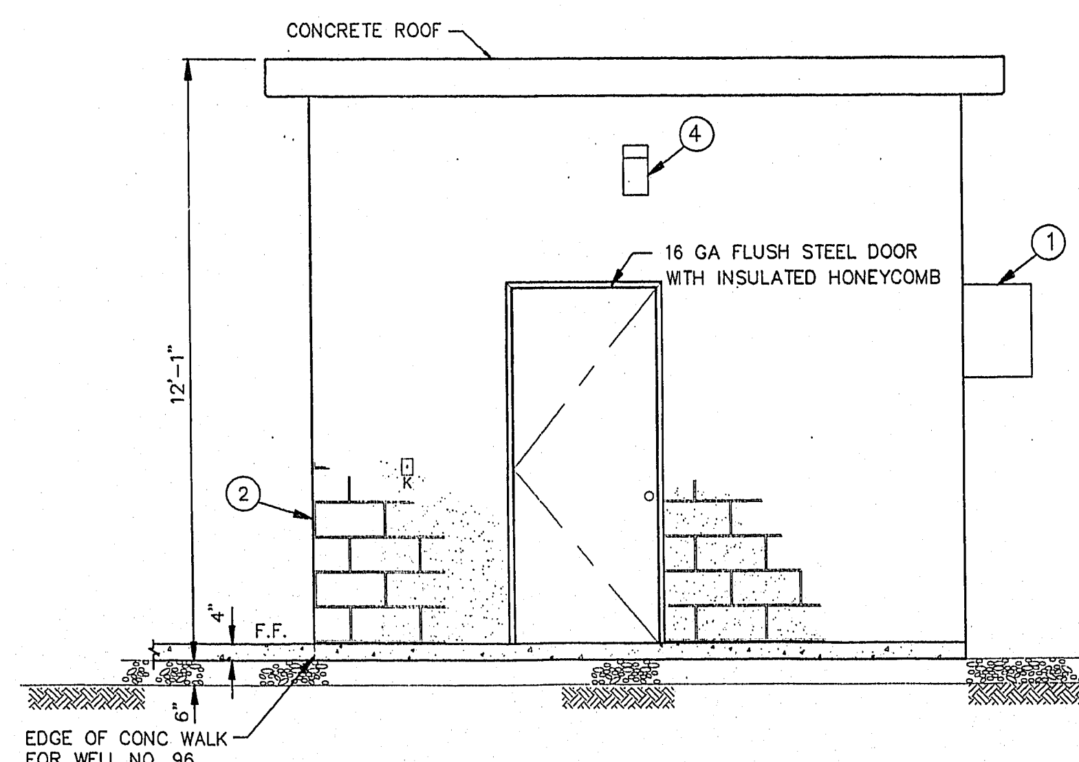
ELEVATION SCALE: 3/8" = 1'-0"
