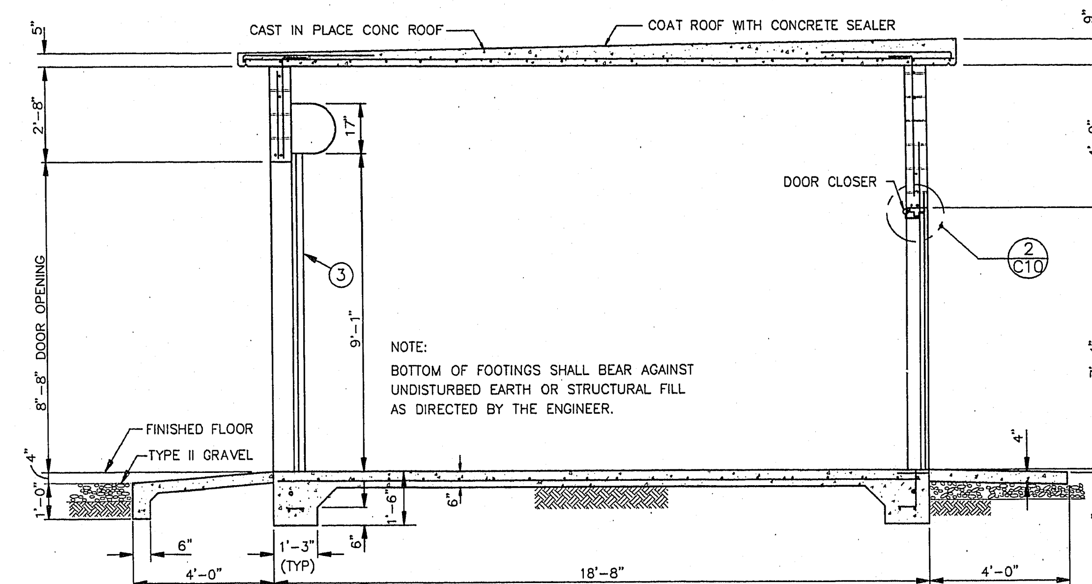
SECTION SCALE: 3/8" = 1'-0"
