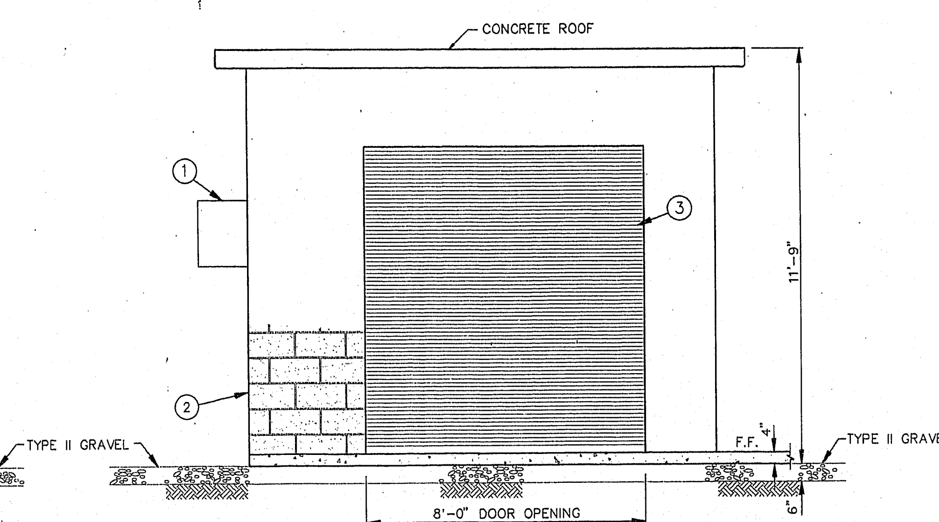
ELEVATION SCALE: 3/8" = 1'-0"
