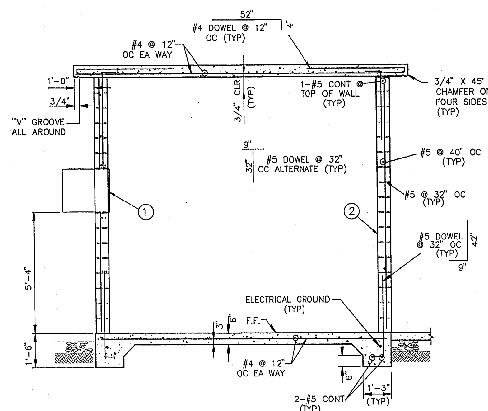
SECTION SCALE: 3/8" = 1'-0"
