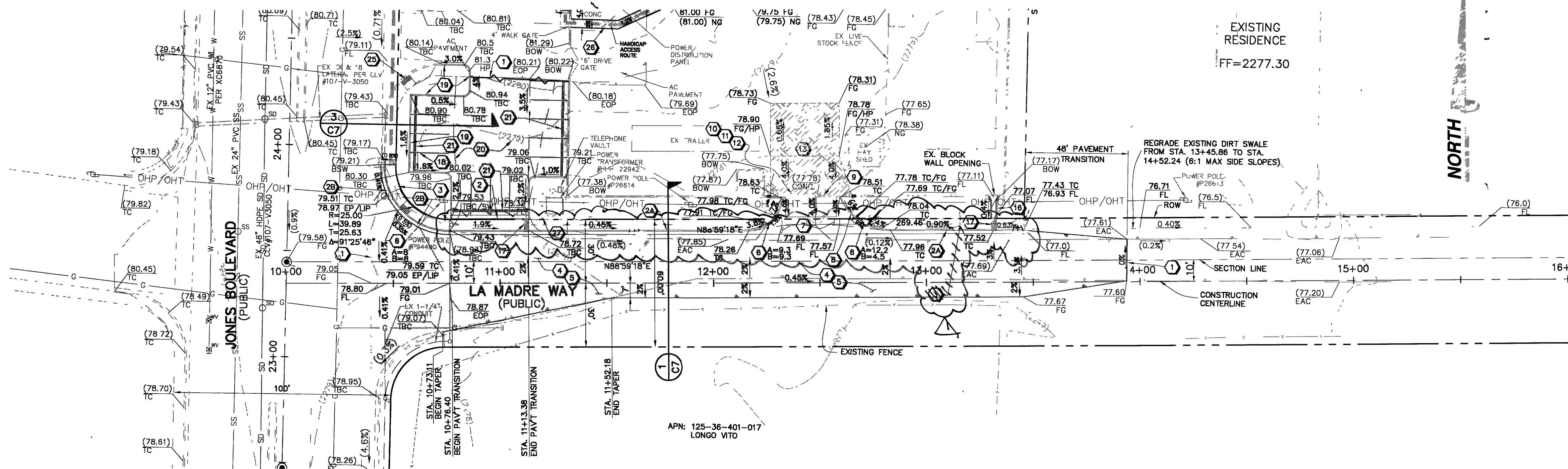
PLAN - LA MADRE WAY SCALE: HORIZ.: 1" = 20'
