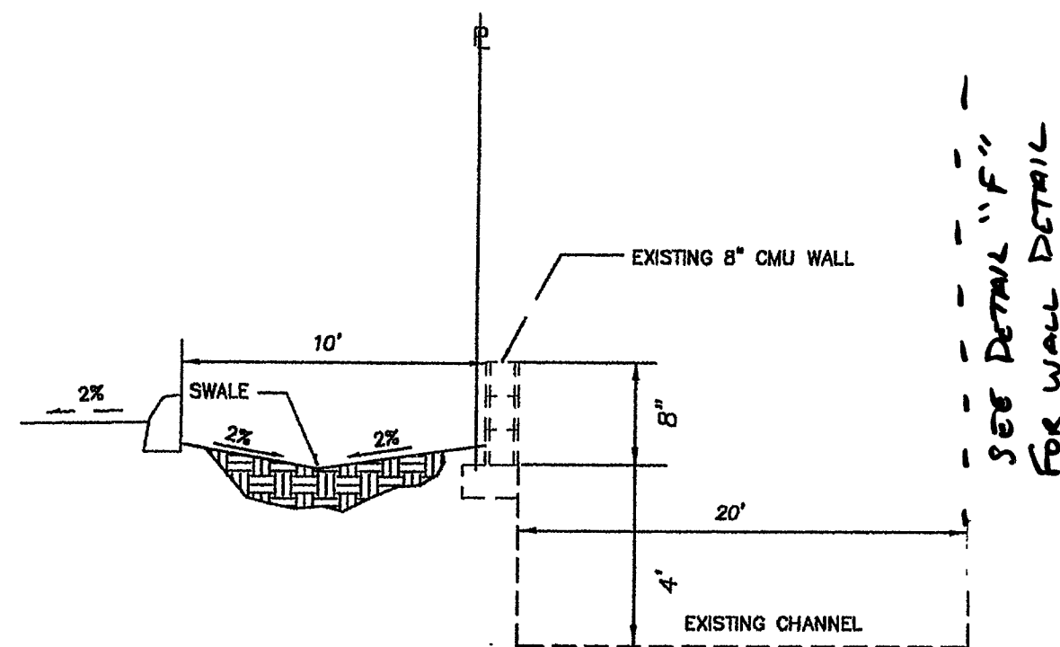
B 8" CMU WALL * See Detail F N.T.S.
