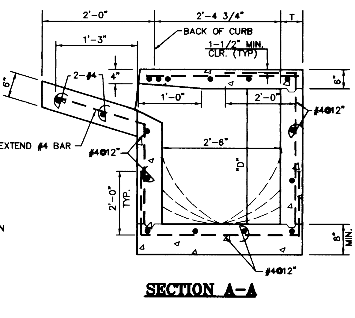
DROP INLET TYPE "CM1" N.T.S.
