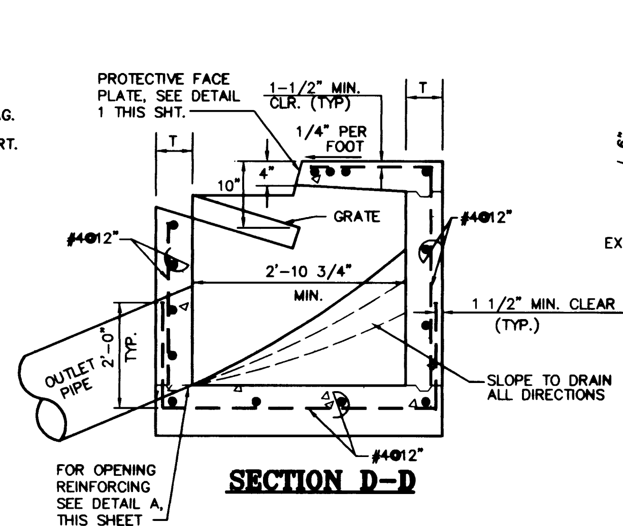
DROP INLET TYPE "DM1" N.T.S.
