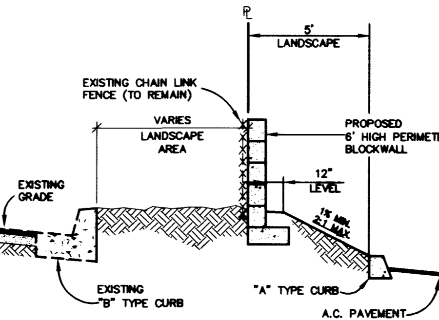
H SECTION SCALE: NO SCALE
