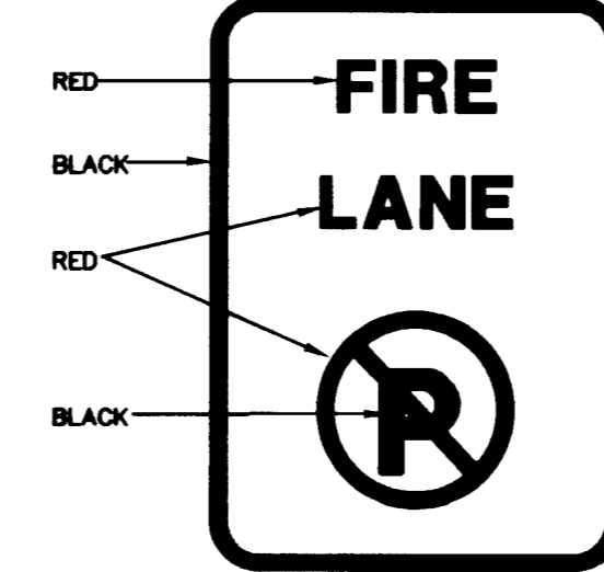
FIRE LANE SIGNAGE SCALE: NO SCALE
