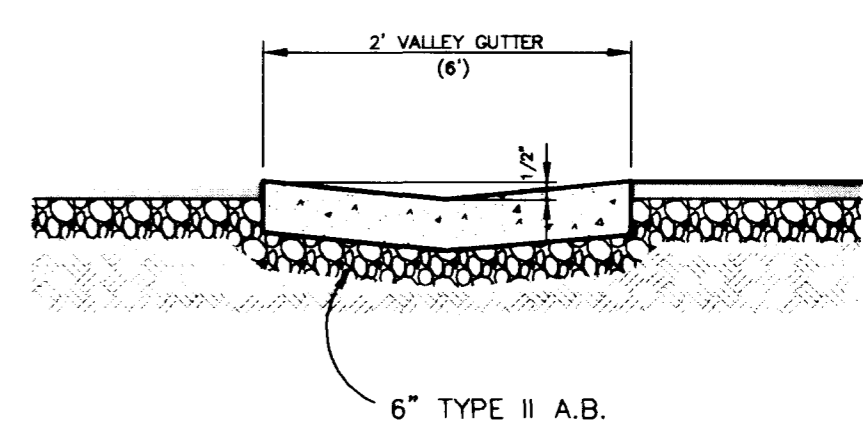
A SECTION SCALE: NO SCALE
