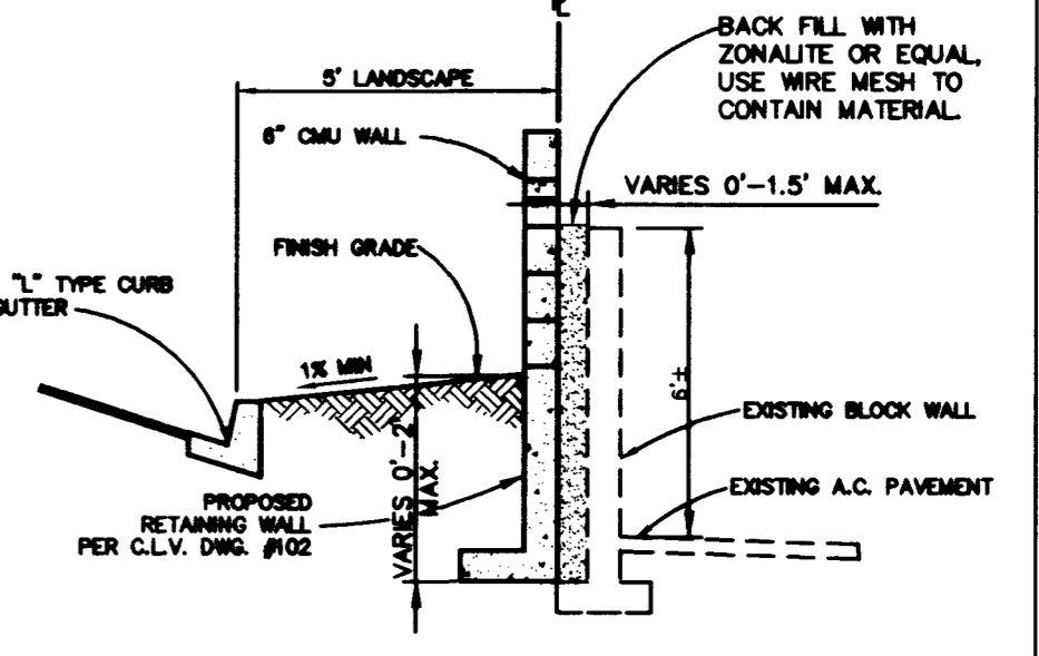
B SECTION SCALE: NO SCALE
