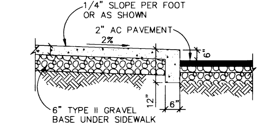
C SECTION SCALE: NO SCALE
