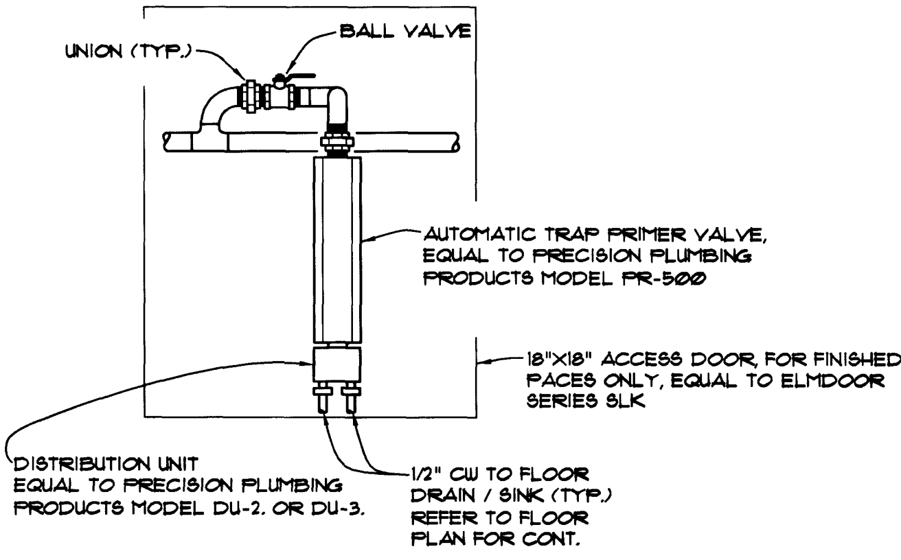
TRAP PRIMER CONNECTION DETAIL 1 NO SCALE
