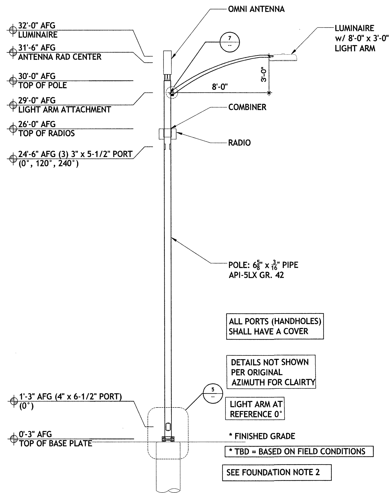
1 POLE ELEVATION
