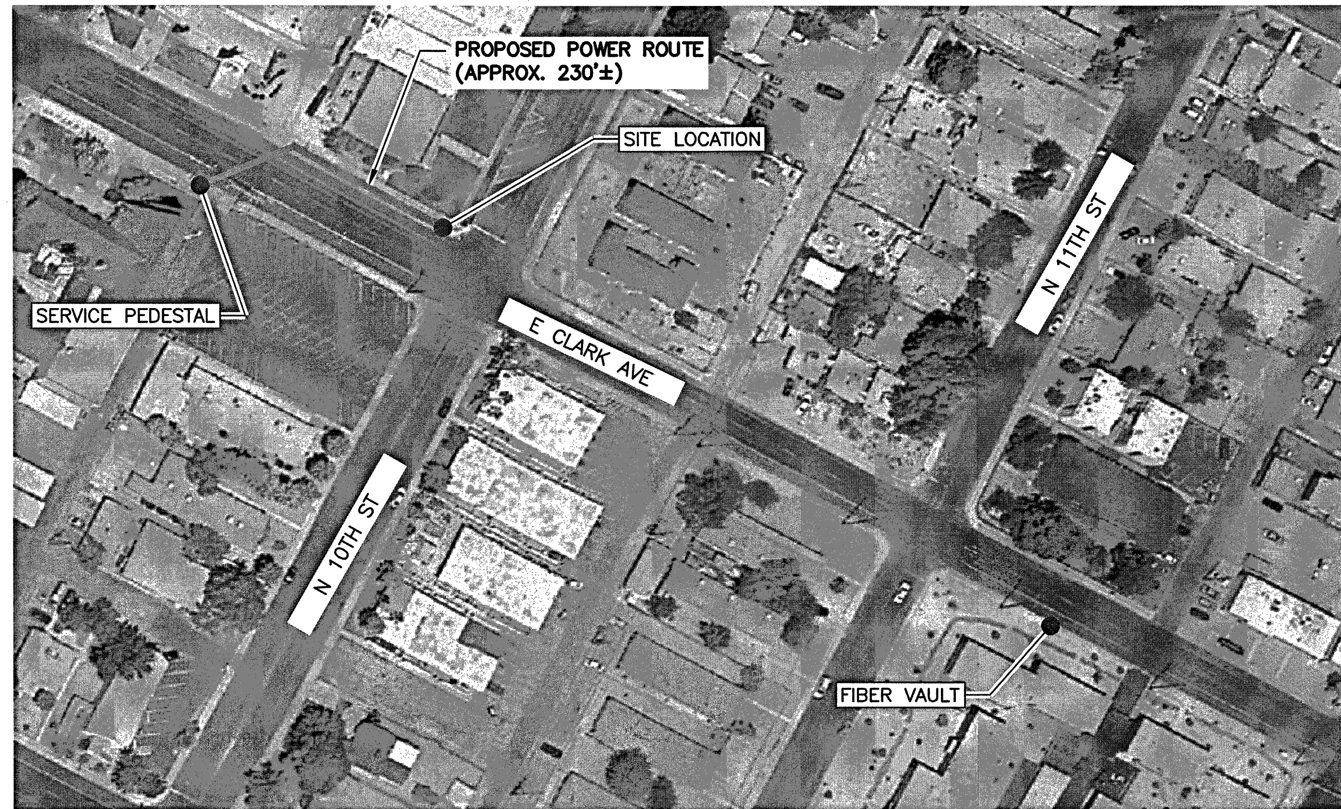
2 AERIAL SITE LOCATION SCALE: N.T.S.
