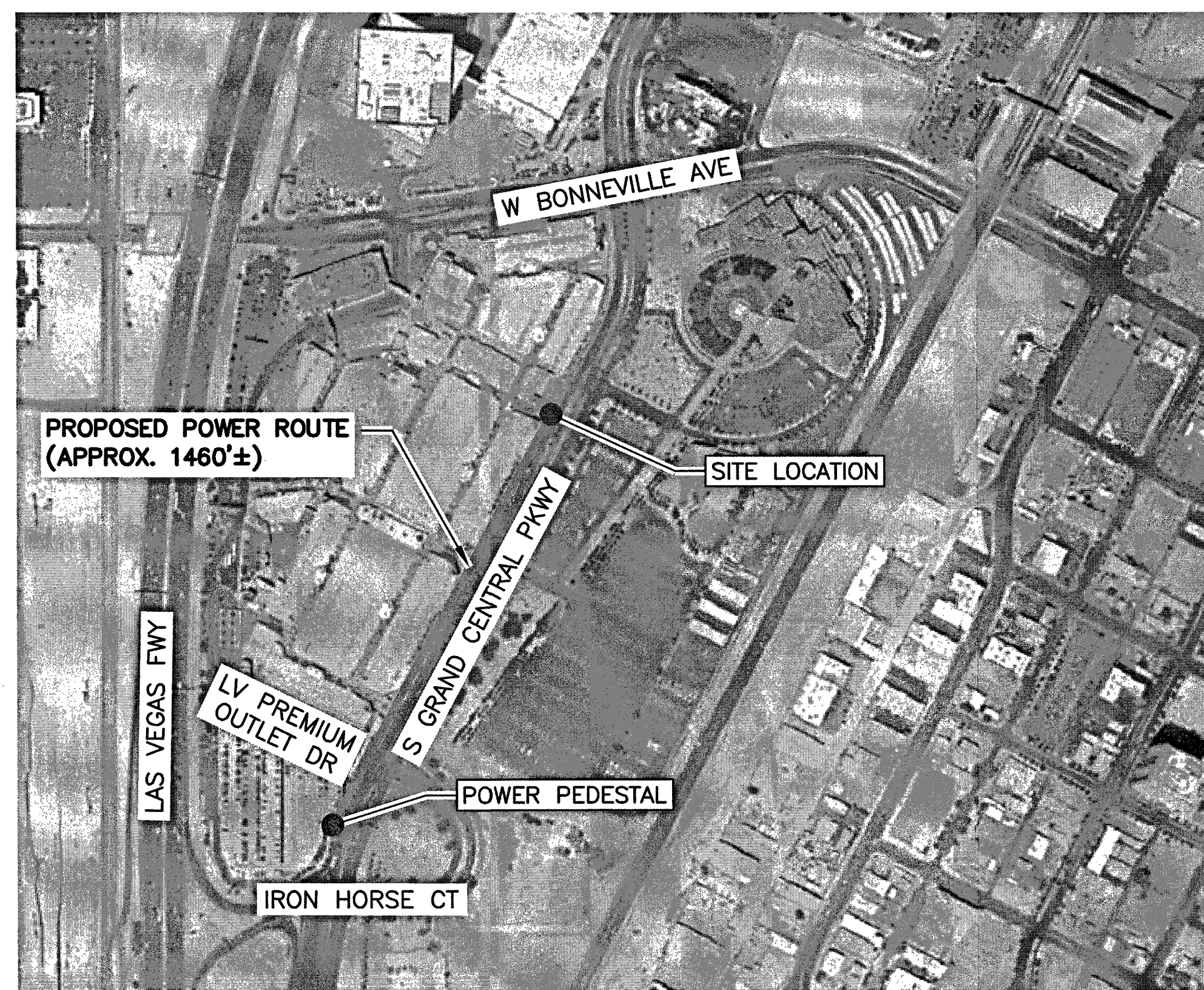
2 AERIAL SITE LOCATION SCALE: N.T.S.
