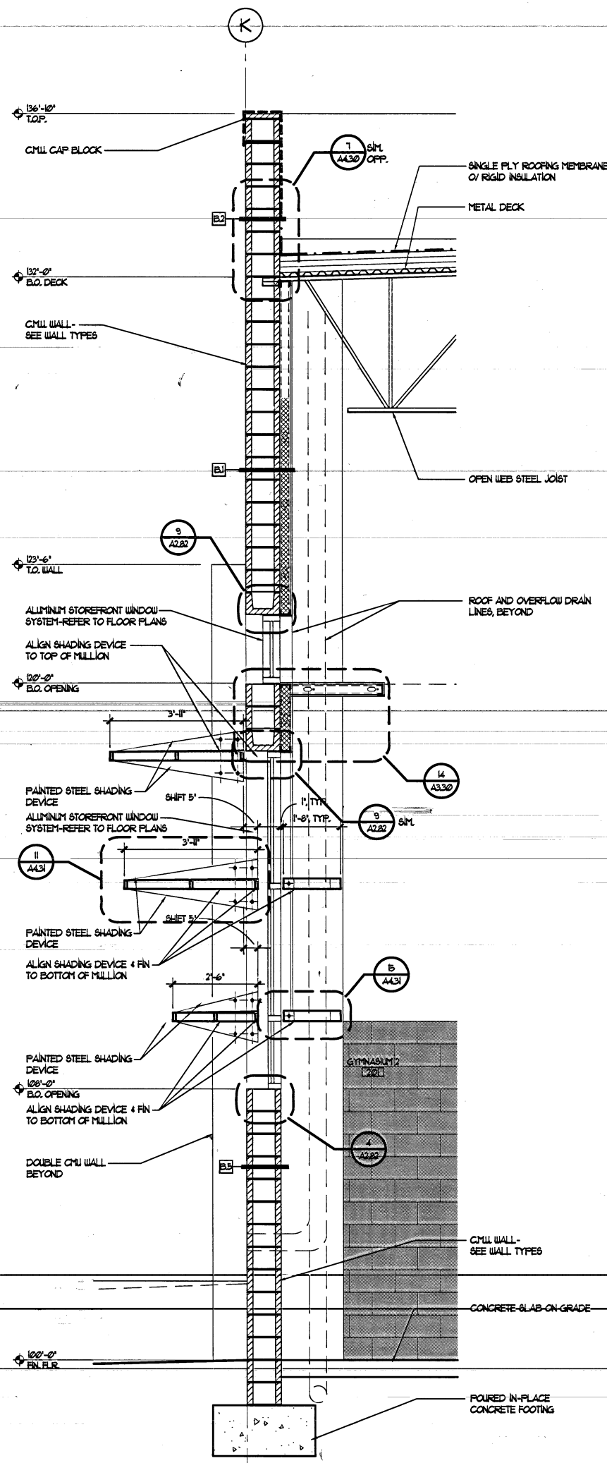
WALL SECTION SCALE: 1/2" = 1'-0"
