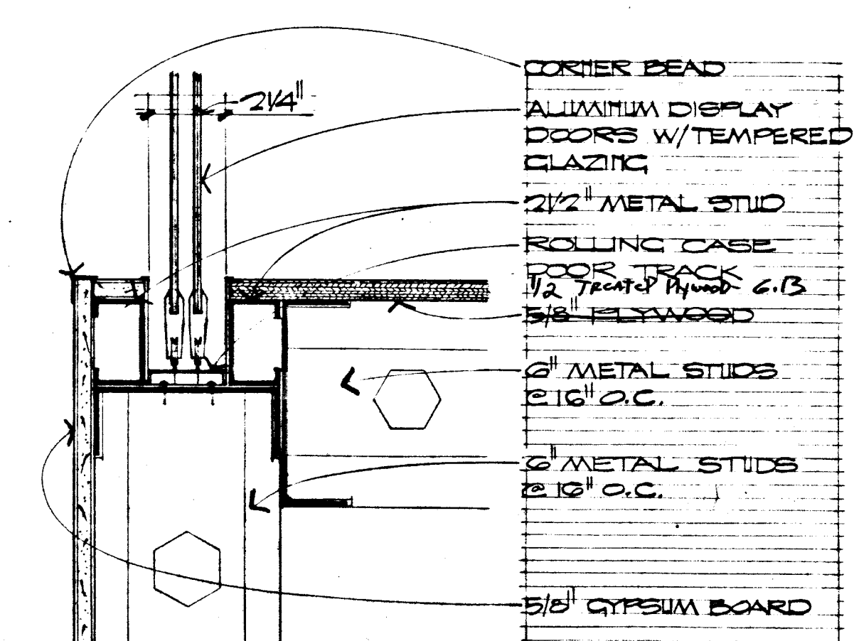
SILL SCALE: 8" = 1'-0" 21 A-7
