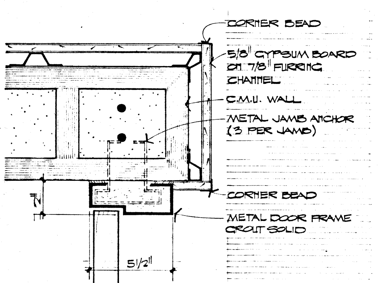
JAMB SCALE: 8" = 1'-0" 28 A-7
