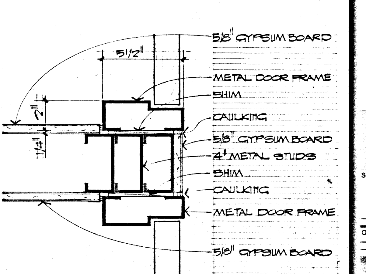
JAMB SCALE: 8" = 1'-0" 30 A-7
