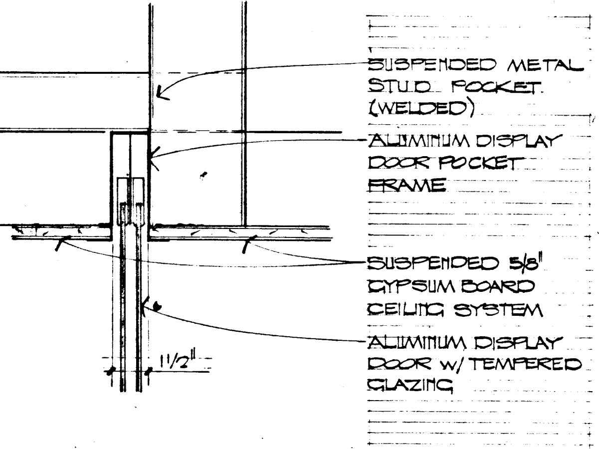
HEAD SCALE: 8" = 1'-0" 15 A-7
