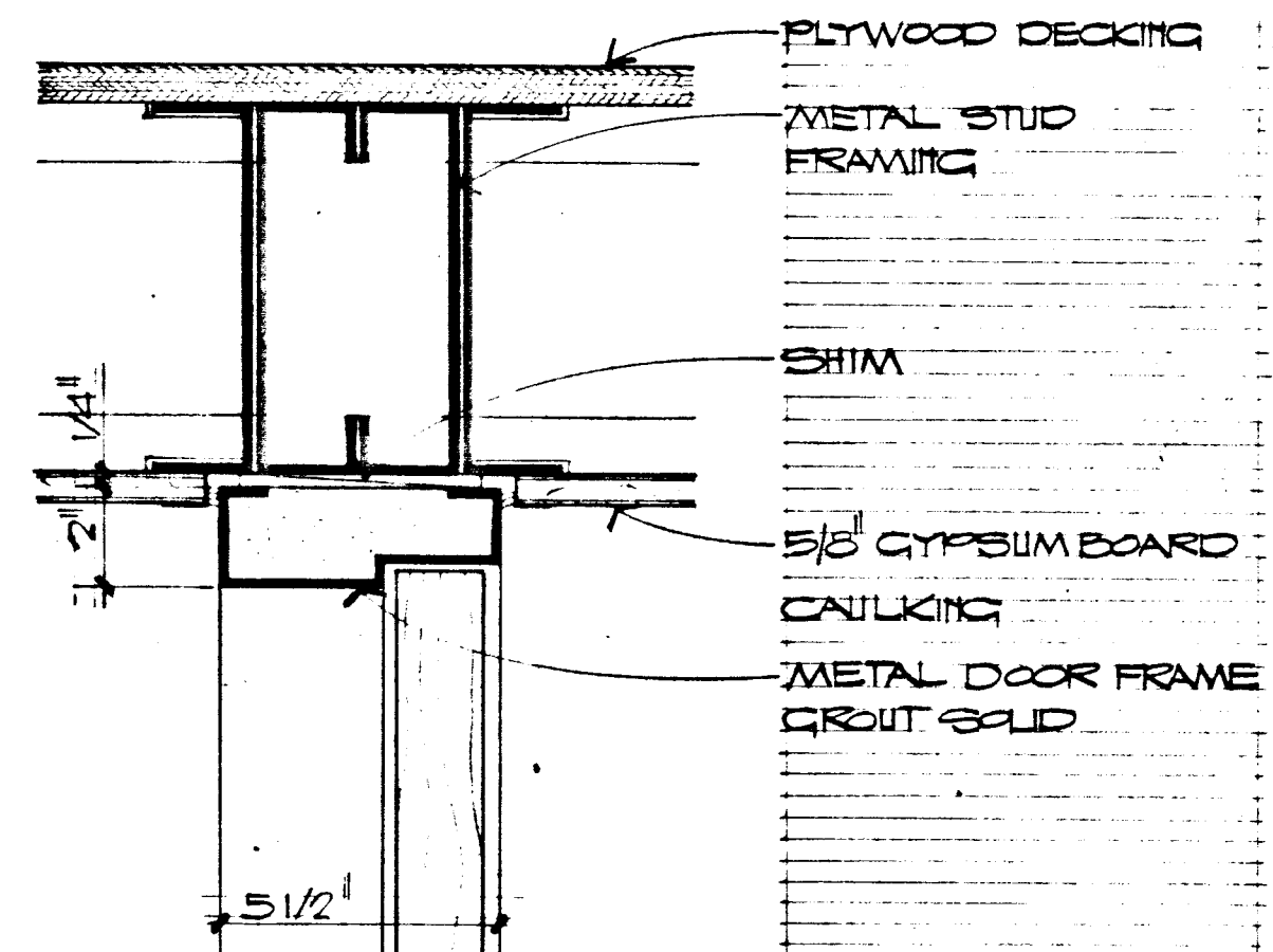
HEAD SCALE: 8" = 1'-0" 14 A-7
