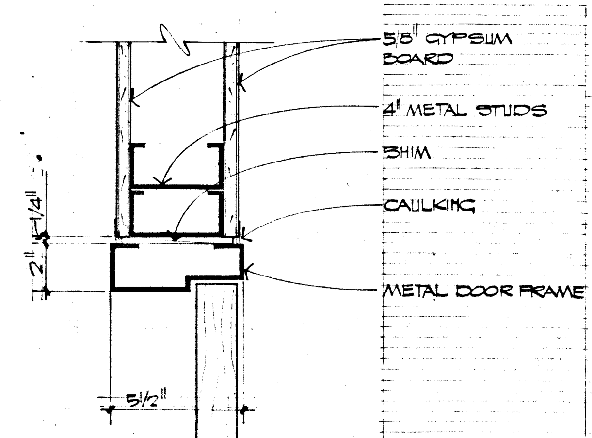
JAMB SCALE: 8" = 1'-0" 25 A-7
