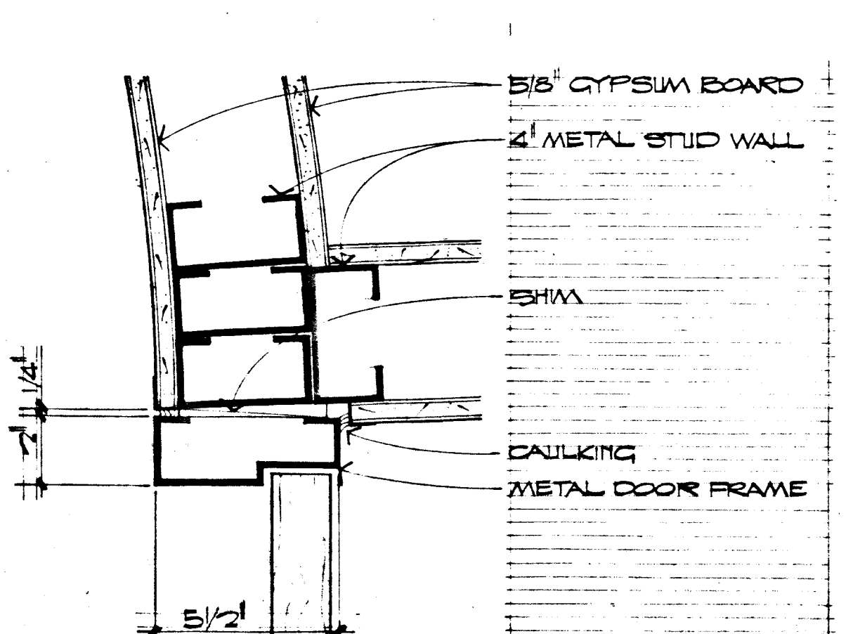
JAMB SCALE: 8" = 1'-0" 22 A-7
