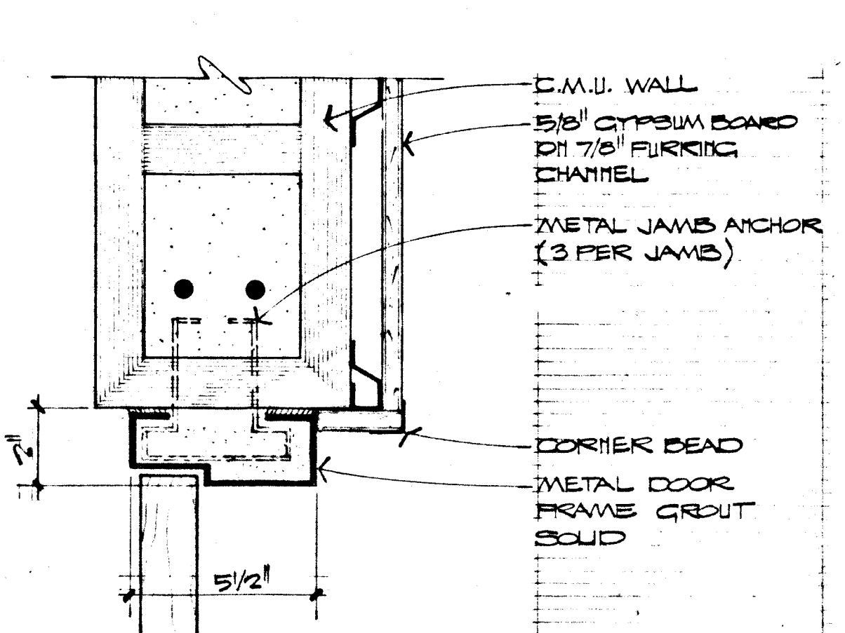
JAMB SCALE: 8" = 1'-0" 29 A-7
