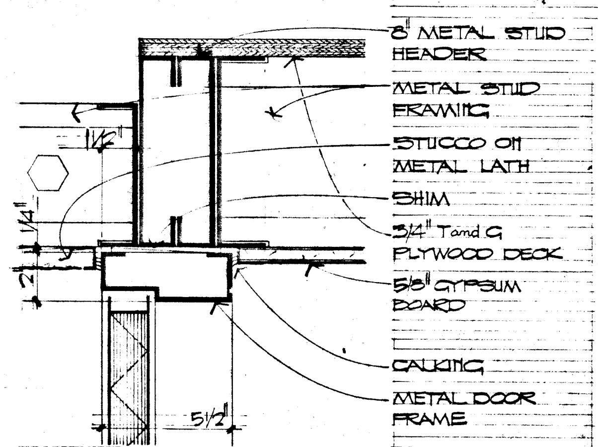
HEAD SCALE: 8" = 1'-0" 2 A-7
