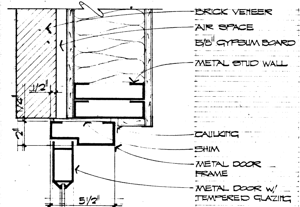
JAMB SCALE: 8" = 1'-0" 7 A-7
