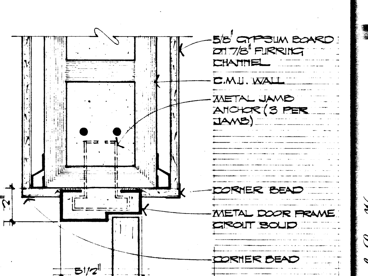
JAMB SCALE: 8" = 1'-0" 24 A-7
