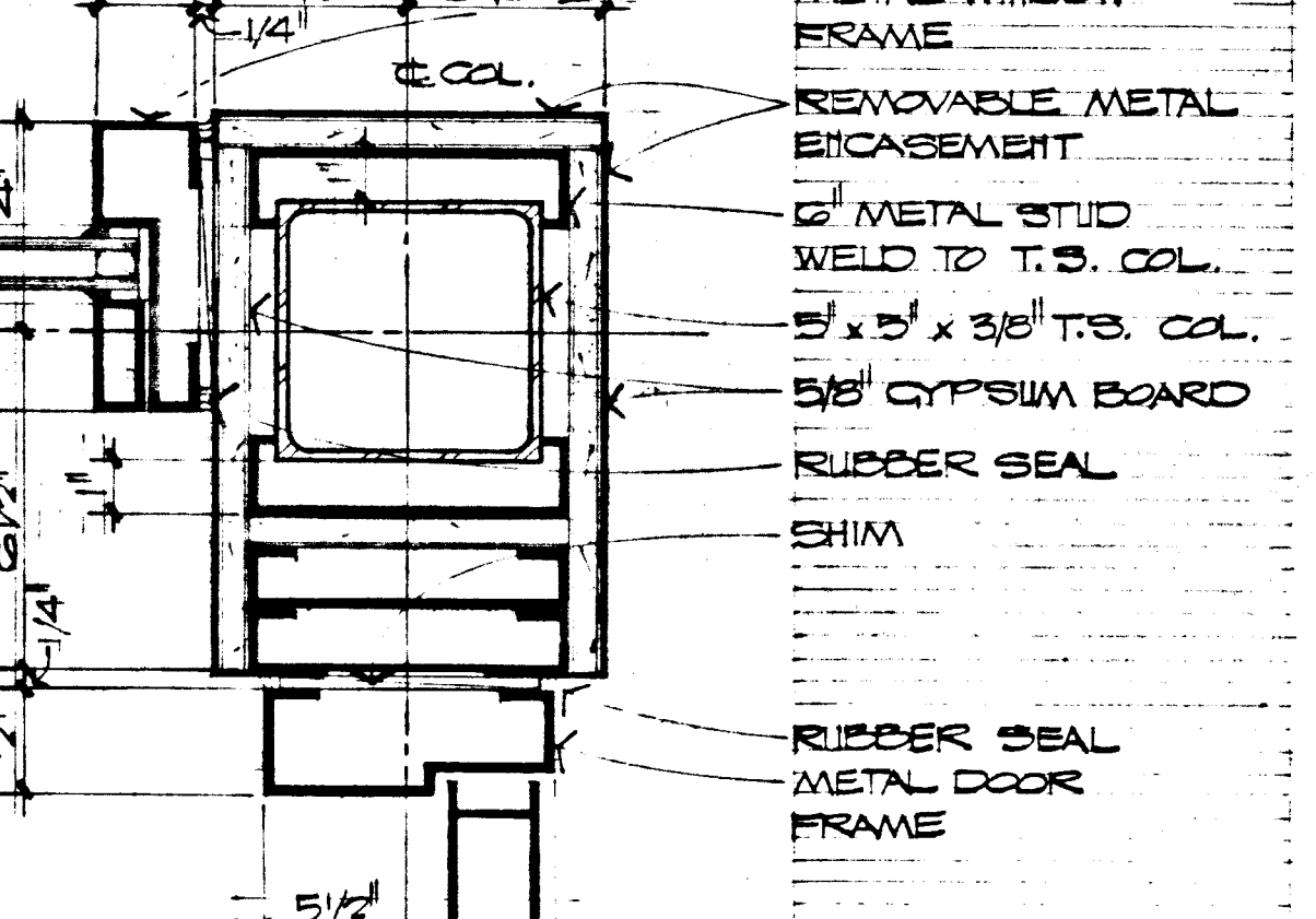
JAMB SCALE: 8" = 1'-0" 10 A-7
