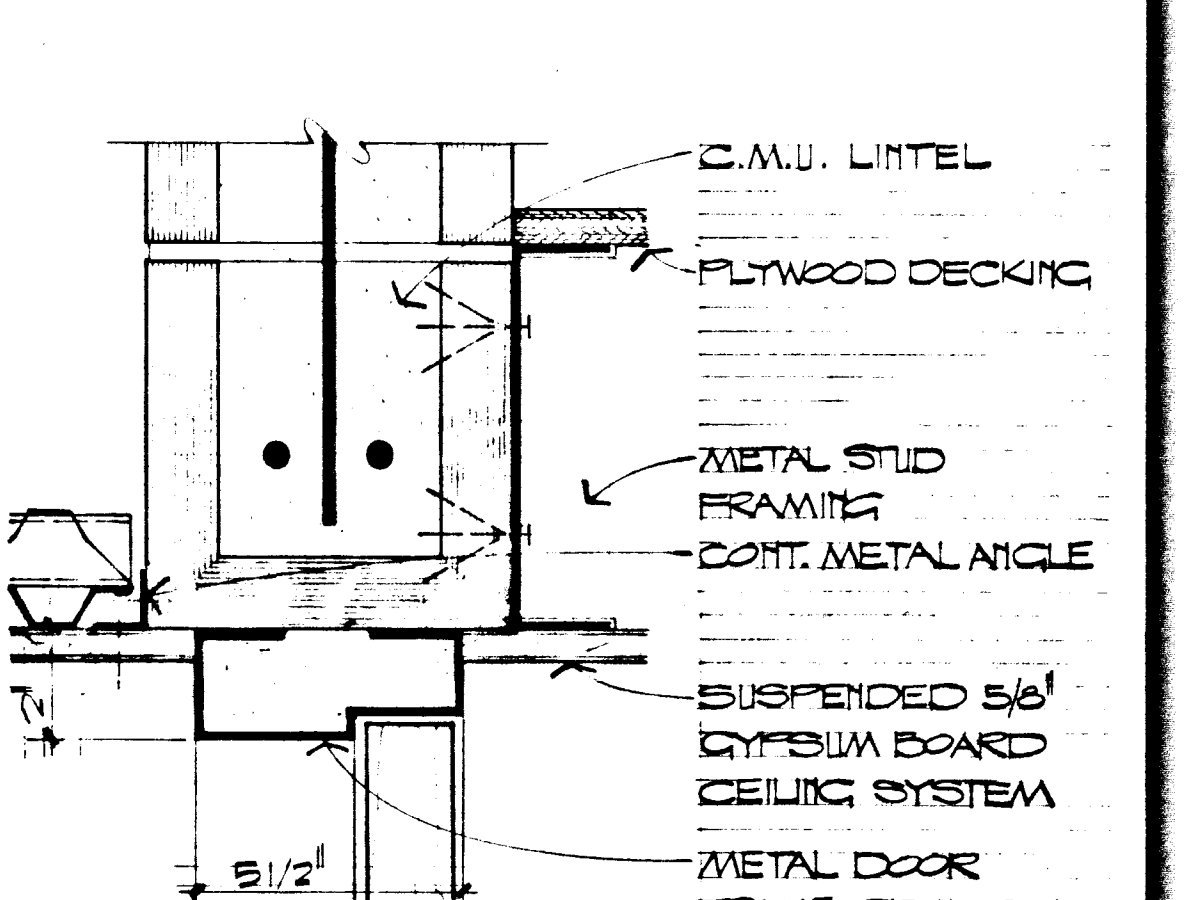
HEAD SCALE: 8" = 1'-0" 18 A-7
