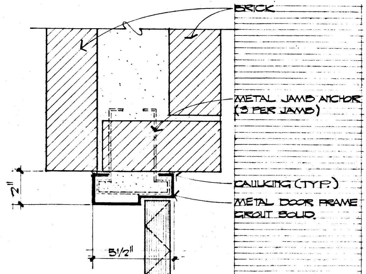
JAMB SCALE: 8" = 1'-0" 26 A-7
