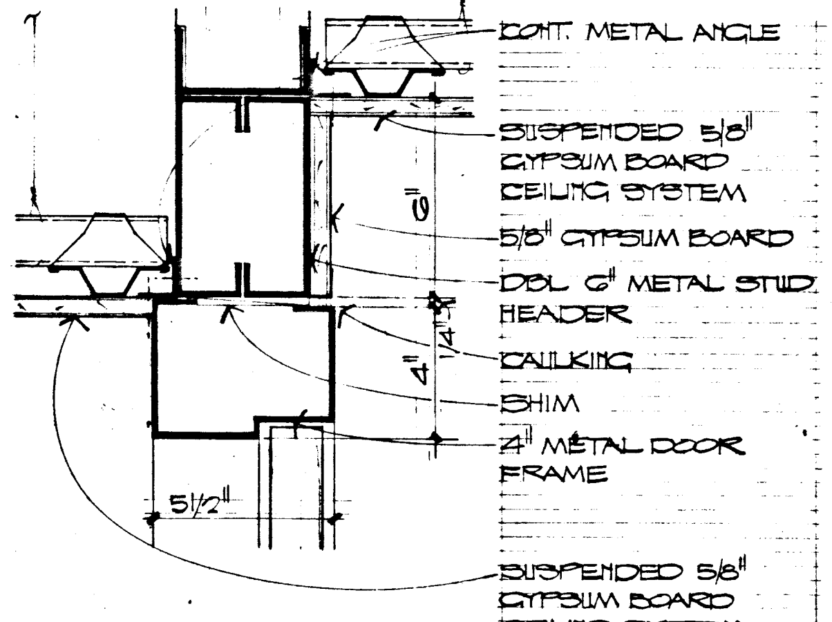
HEAD SCALE: 8" = 1'-0" 16 A-7
