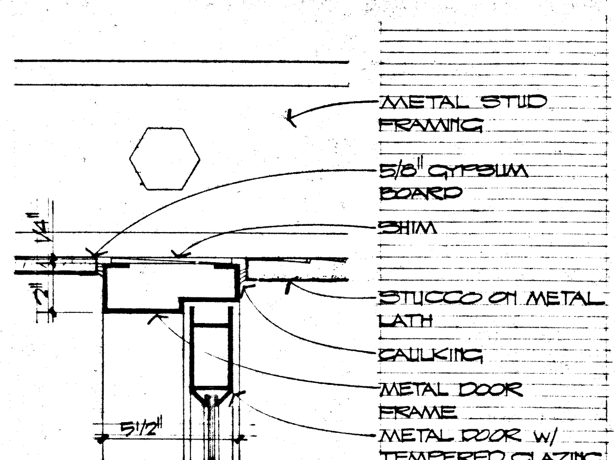
HEAD SCALE: 8" = 1'-0" 3 A-7
