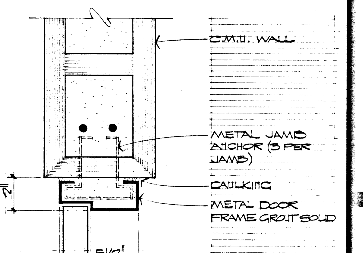
JAMB SCALE: 8" = 1'-0" 12 A-7
