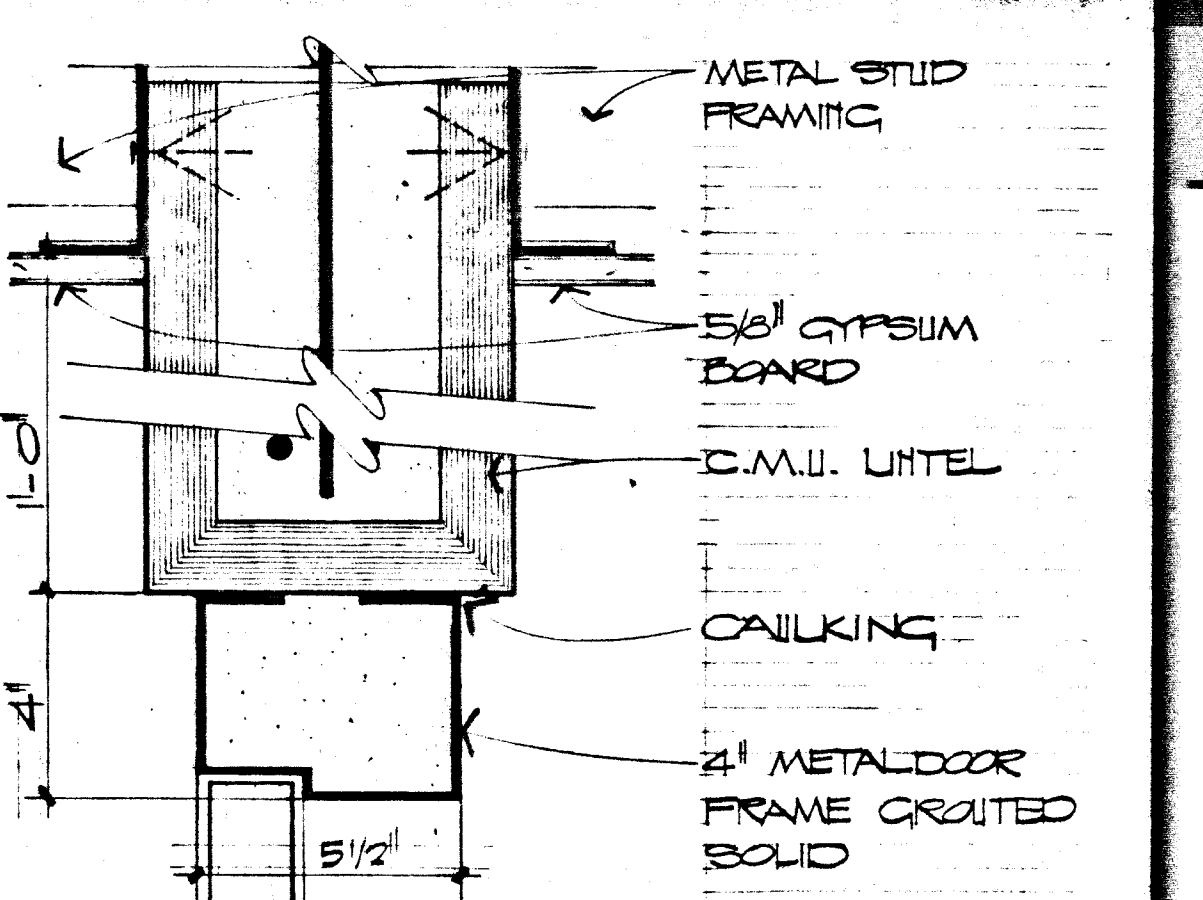
HEAD SCALE: 8" = 1'-0" 6 A-7
