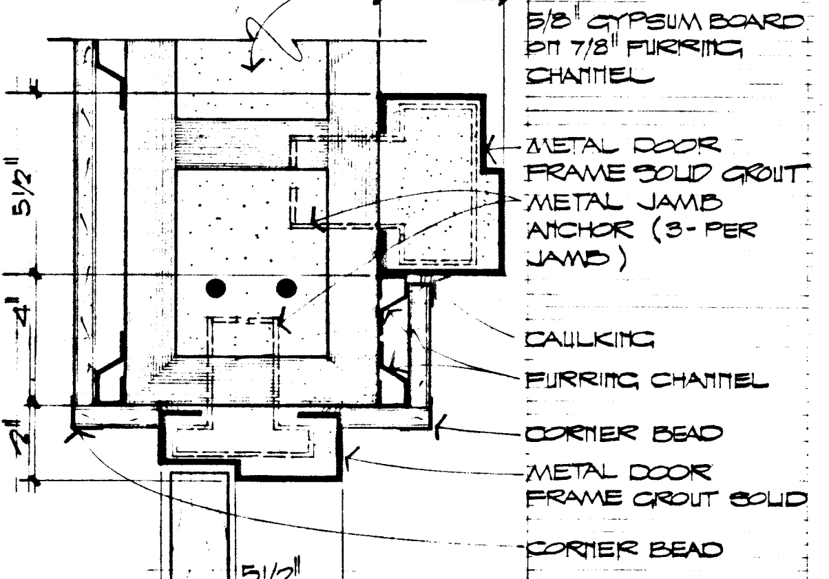
JAMB SCALE: 8" = 1'-0" 11 A-7
