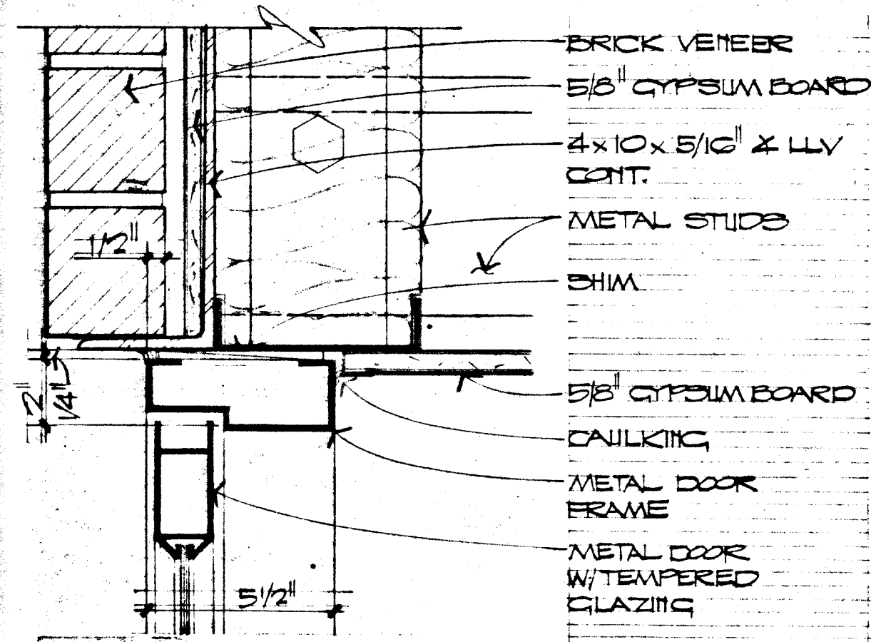
HEAD SCALE: 8" = 1'-0" 1 A-7
