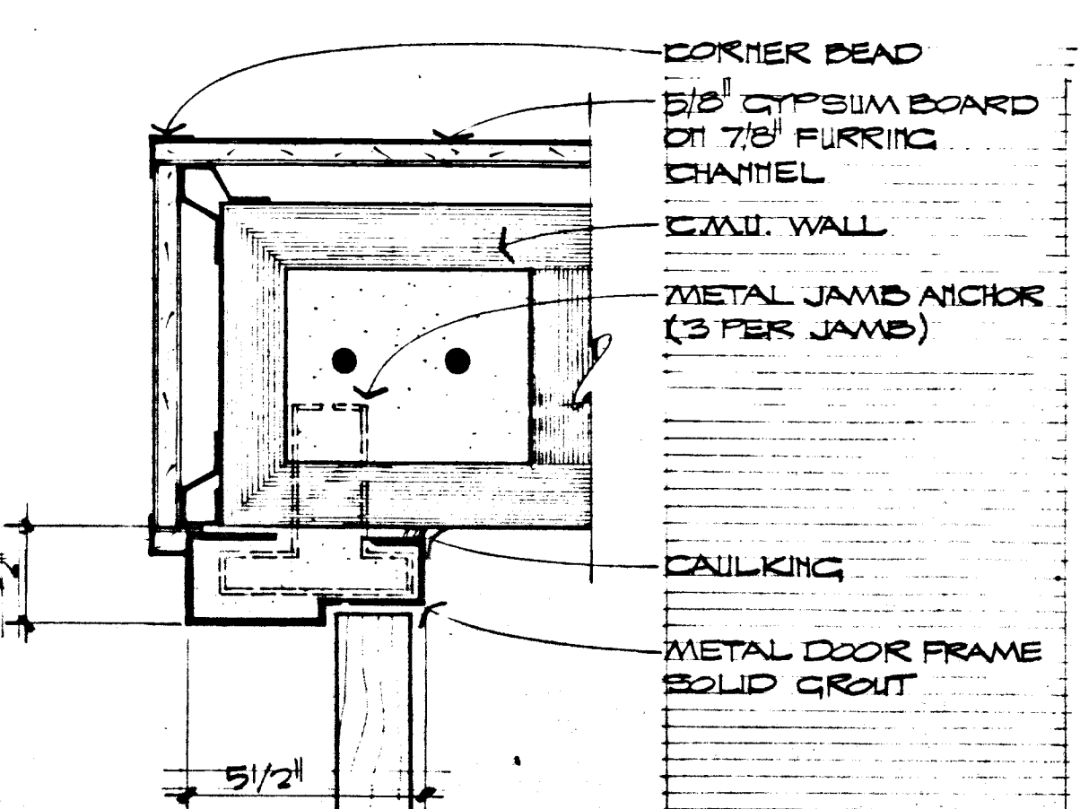
JAMB SCALE: 8" = 1'-0" 20 A-7
