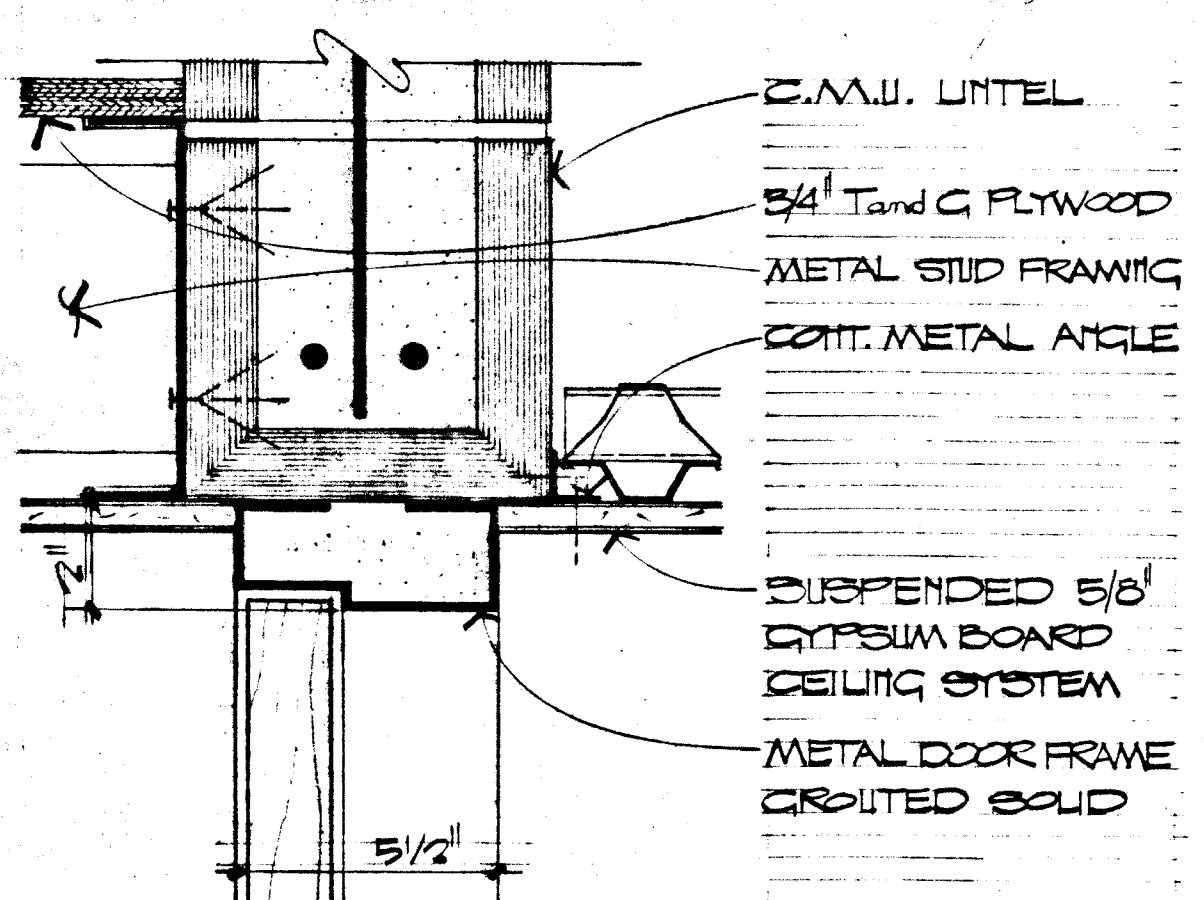
HEAD SCALE: 8" = 1'-0" 5 A-7
