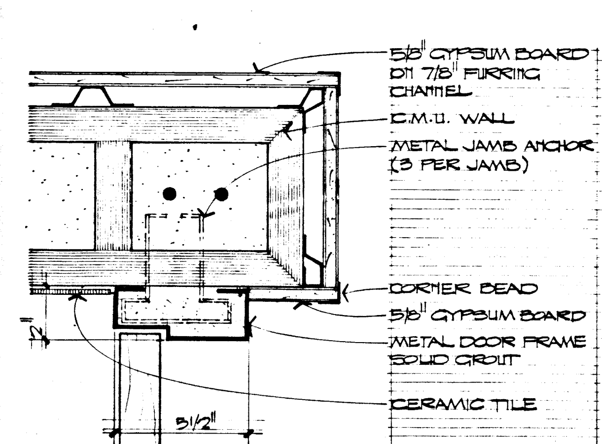
JAMB SCALE: 8" = 1'-0" 19 A-7
