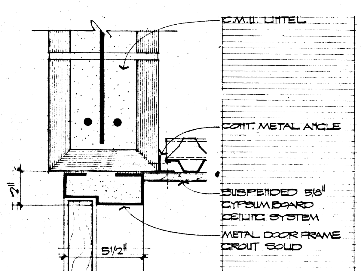
HEAD SCALE: 8" = 1'-0" 27 A-7
