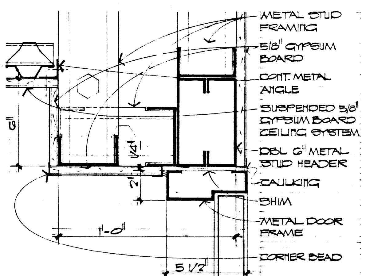
HEAD SCALE: 8" = 1'-0" 17 A-7
