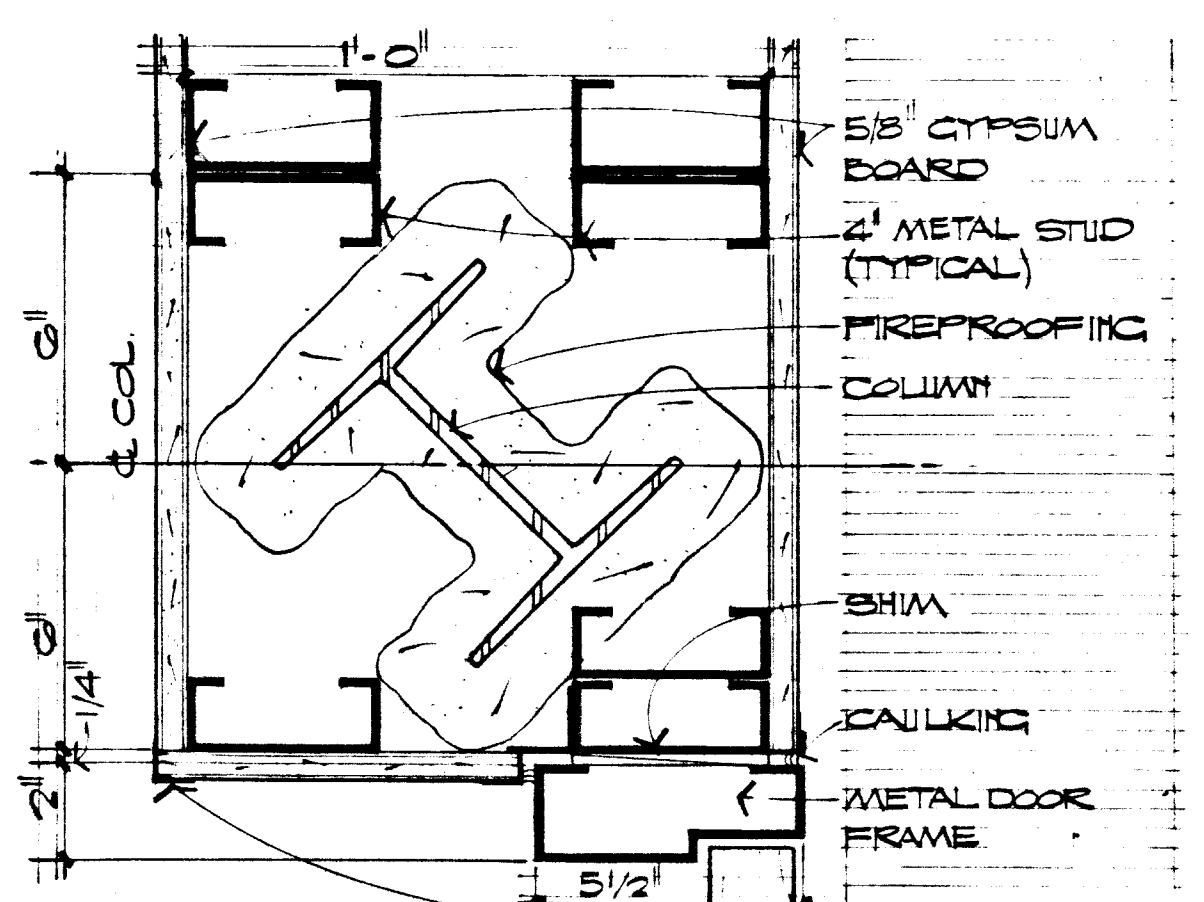
JAMB SCALE: 8" = 1'-0" 23 A-7
