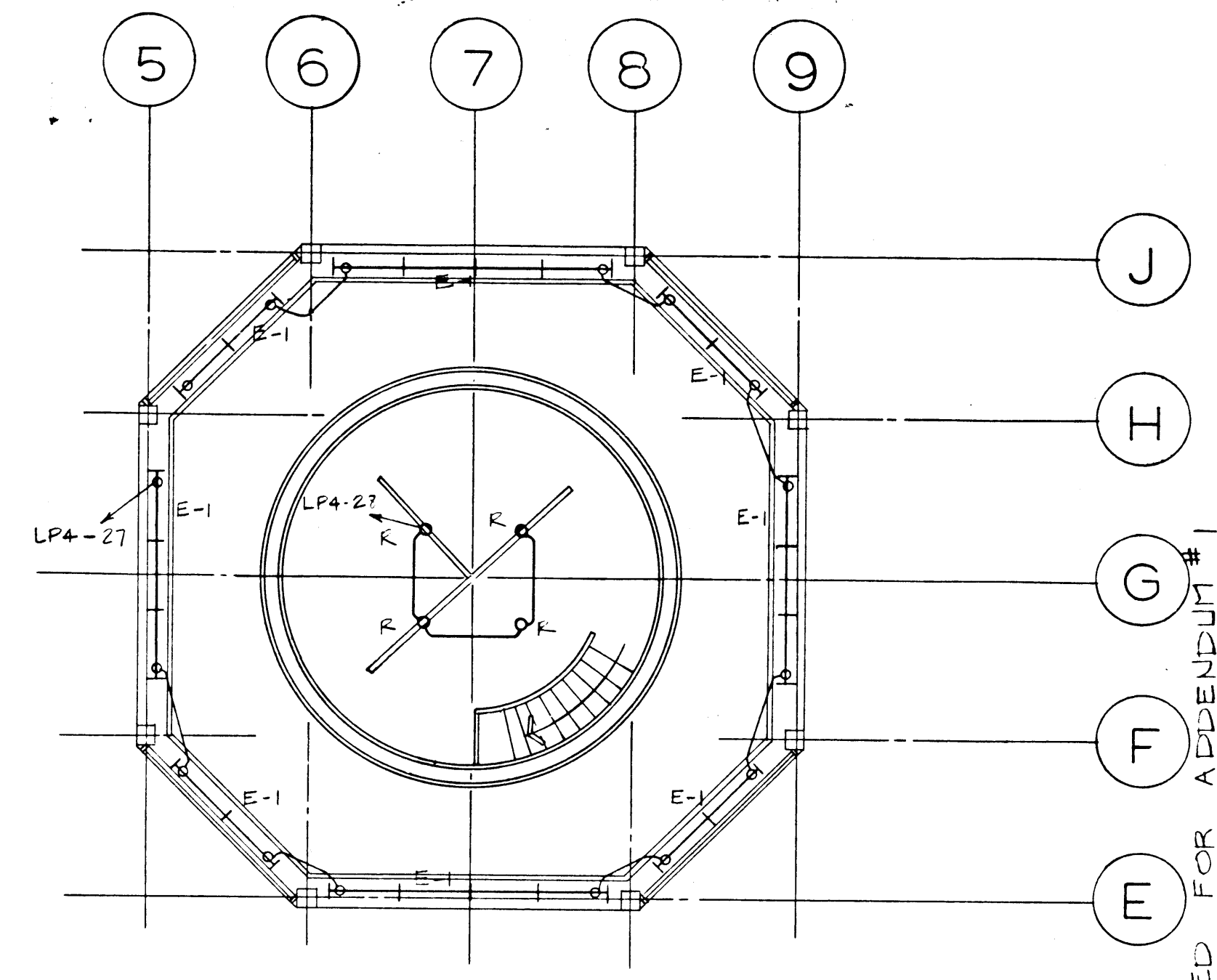
UPPER LEVEL SCALE: 1/8" = 1'-0"
