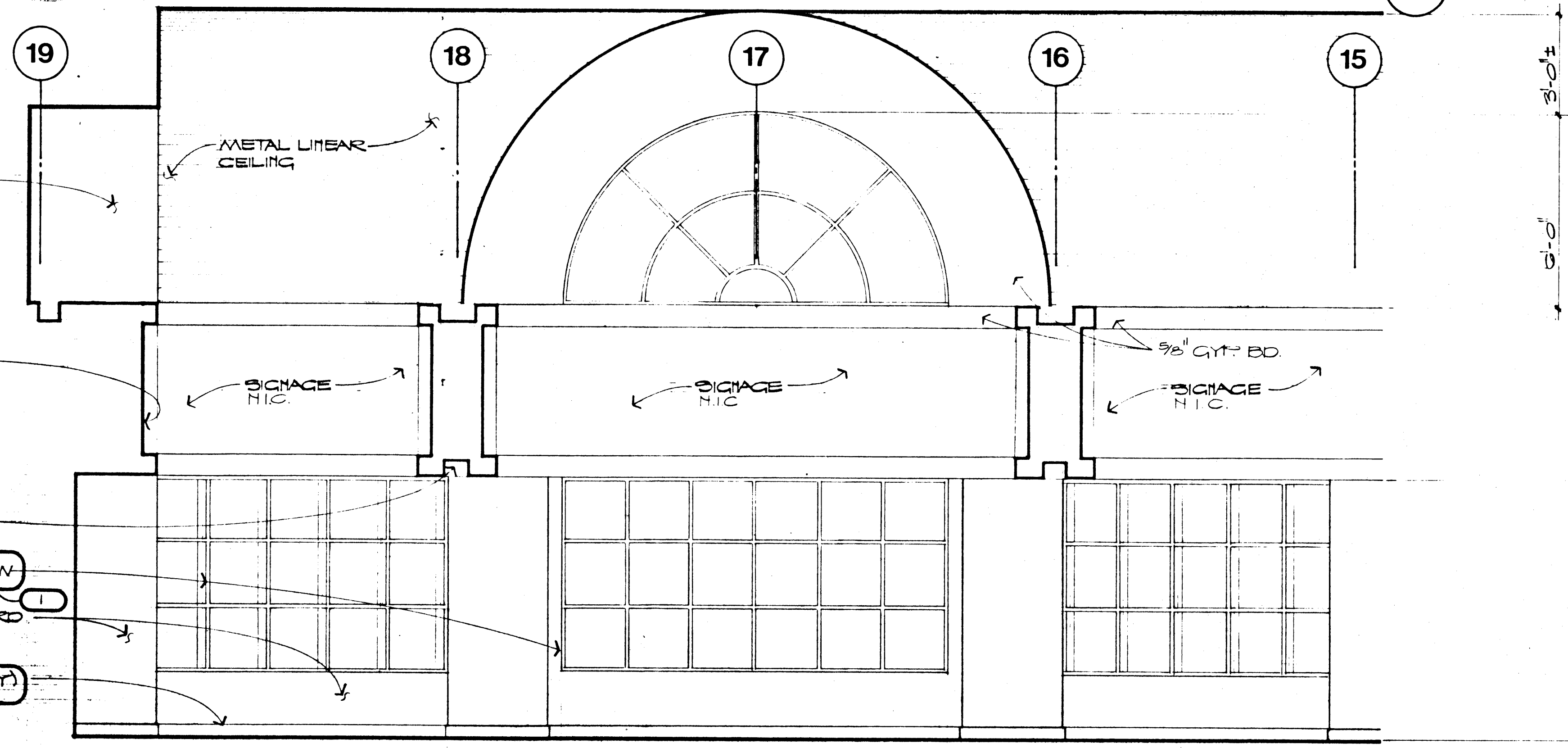
LOBBY #5 SCALE: 3/8" = 1'-0"
