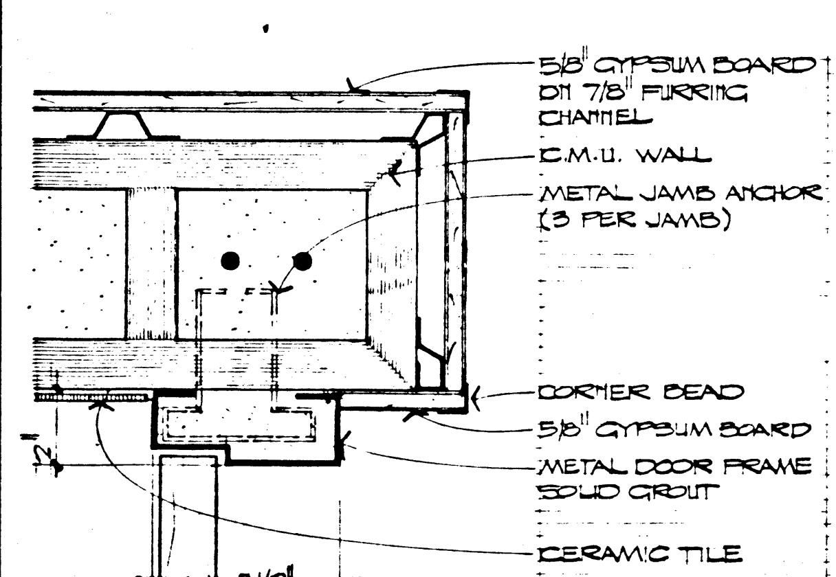
JAMB SCALE: 8" = 1'-0" 19 A-7
