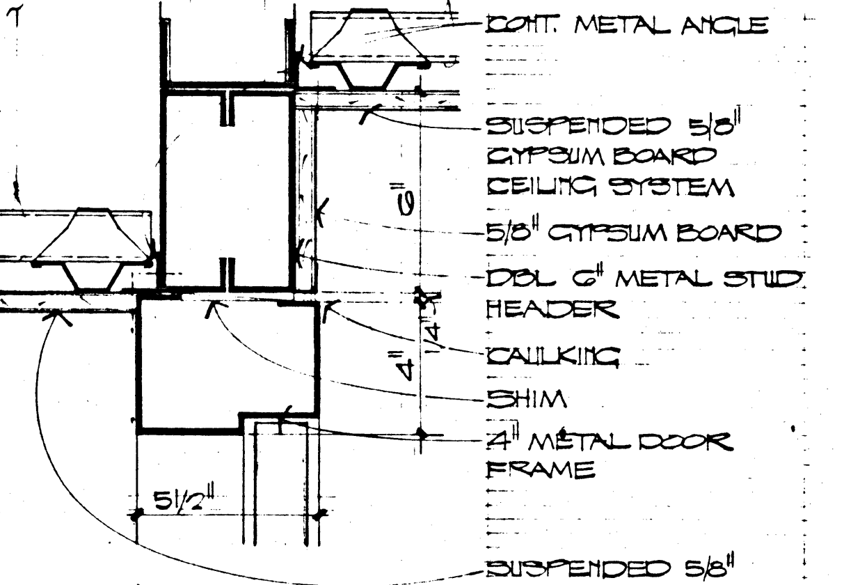
HEAD SCALE: 8" = 1'-0" 16 A-7
