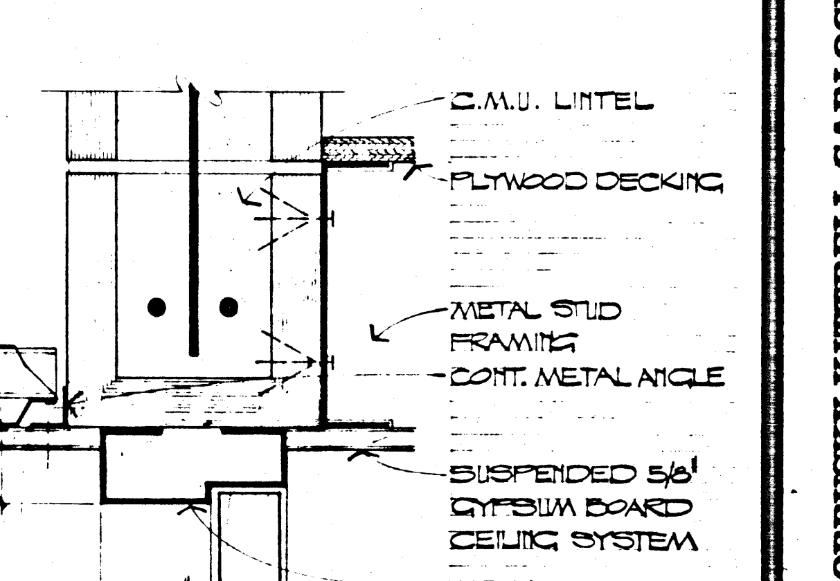
HEAD SCALE: 8" = 1'-0" 18 A-7
