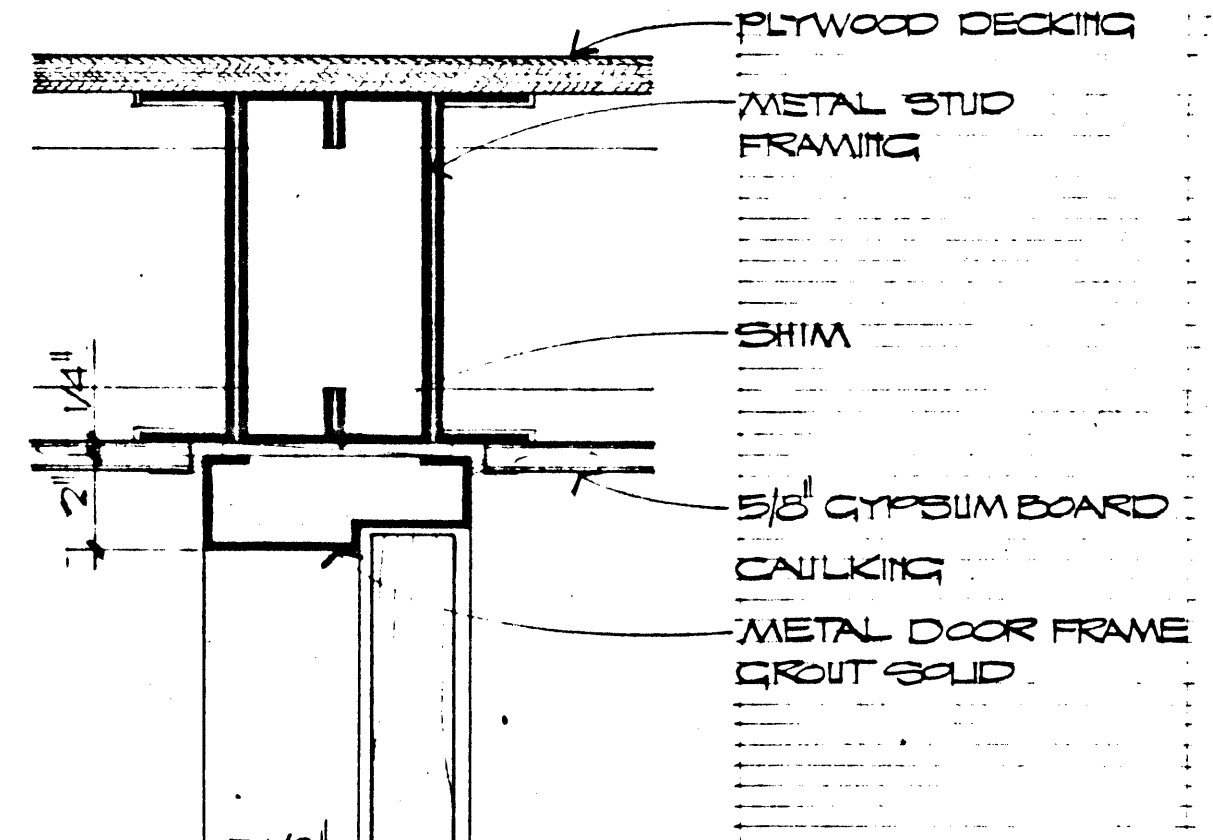
HEAD SCALE: 8" = 1'-0" 14 A-7
