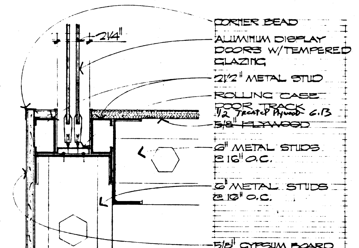
SILL SCALE: 8" = 1'-0" 21 A-7
