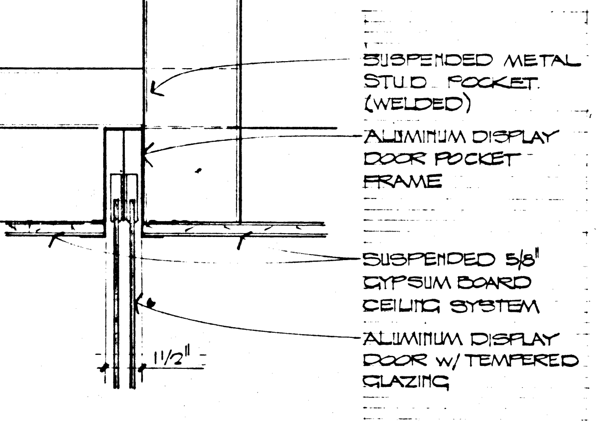
HEAD SCALE: 8" = 1'-0" 15 A-7
