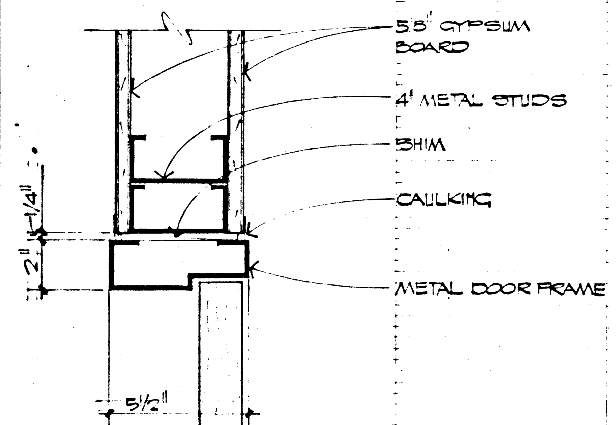
JAMB SCALE: 8" = 1'-0" 25 A-7
