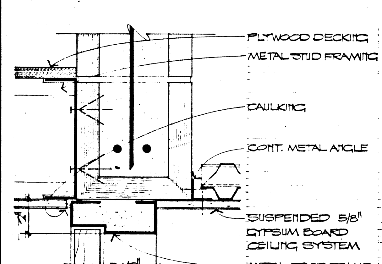
HEAD SCALE: 8" = 1'-0" 13 A-7
