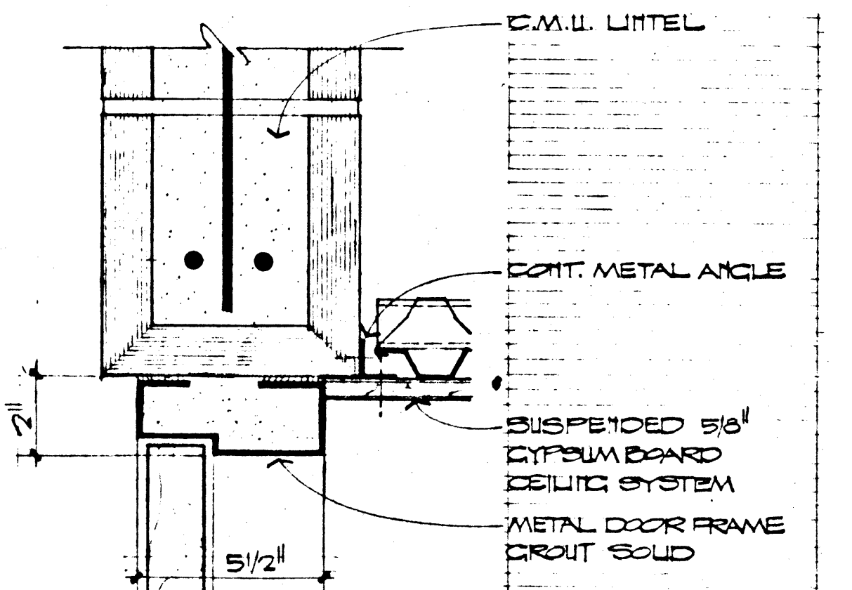
HEAD SCALE: 8" = 1'-0" 27 A-7
