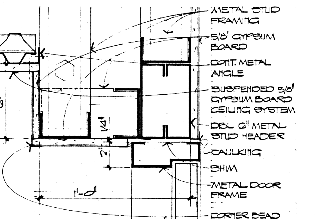
HEAD SCALE: 8" = 1'-0" 17 A-7
