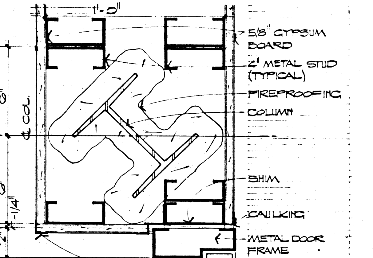
JAMB SCALE: 8" = 1'-0" 23 A-7
