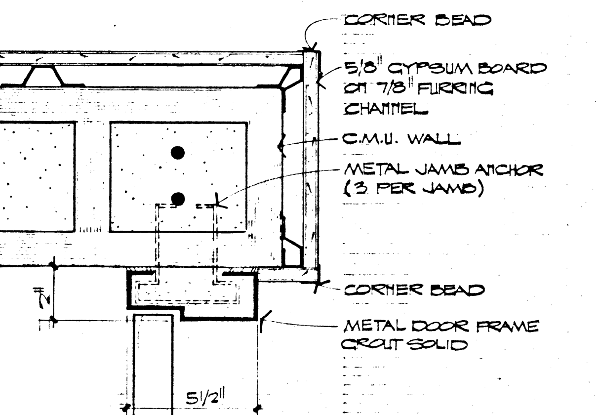
JAMB SCALE: 8" = 1'-0" 28 A-7
