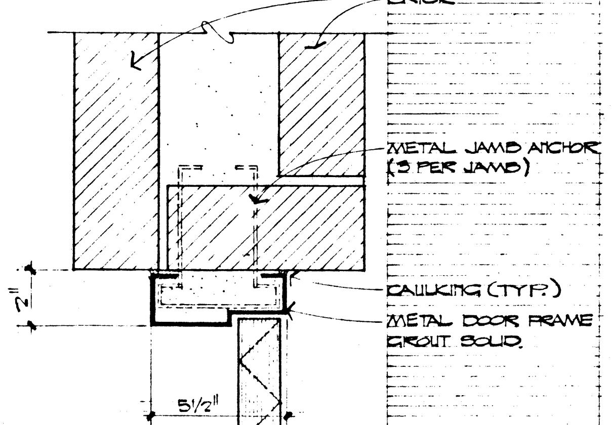
JAMB SCALE: 8" = 1'-0" 26 A-7
