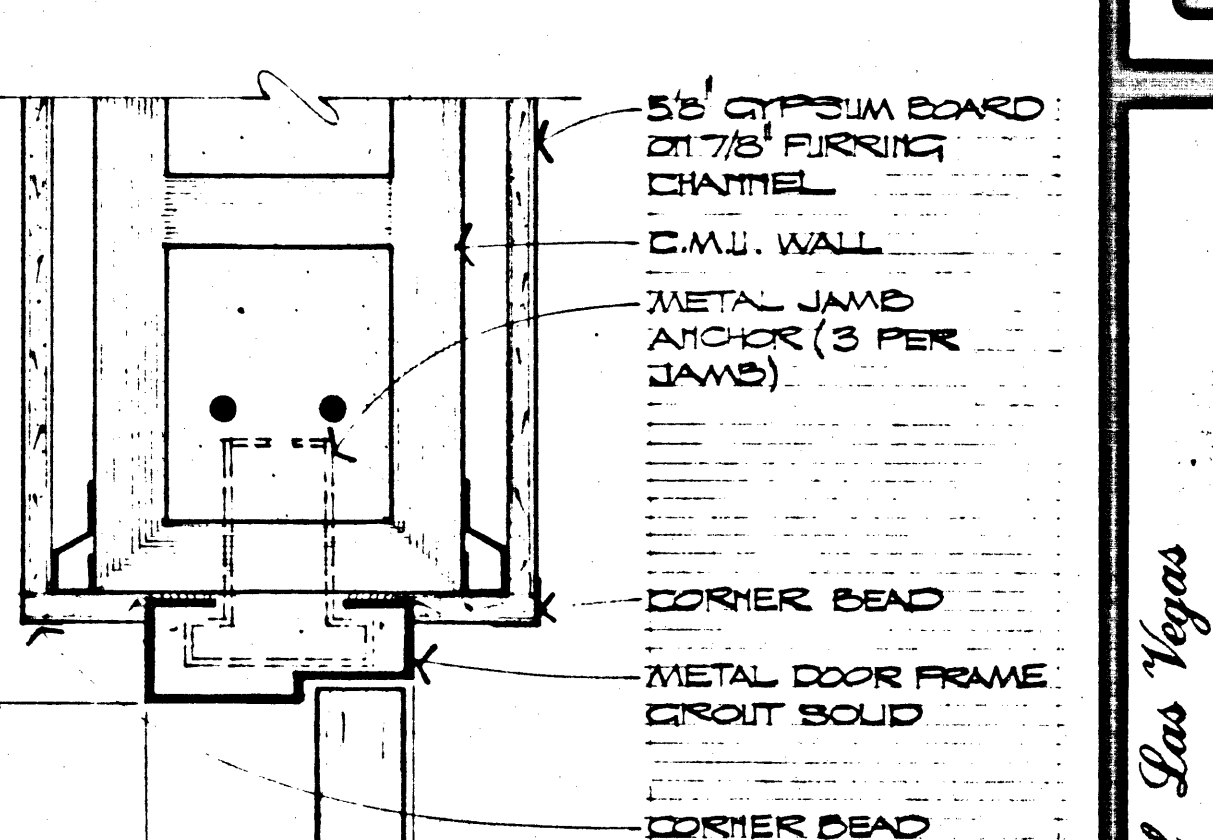
JAMB SCALE: 8" = 1'-0" 24 A-7
