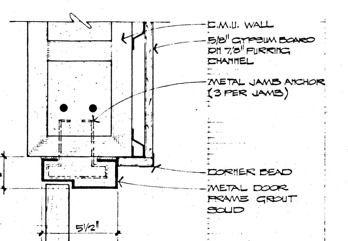
JAMB SCALE: 8" = 1'-0" 29 A-7
