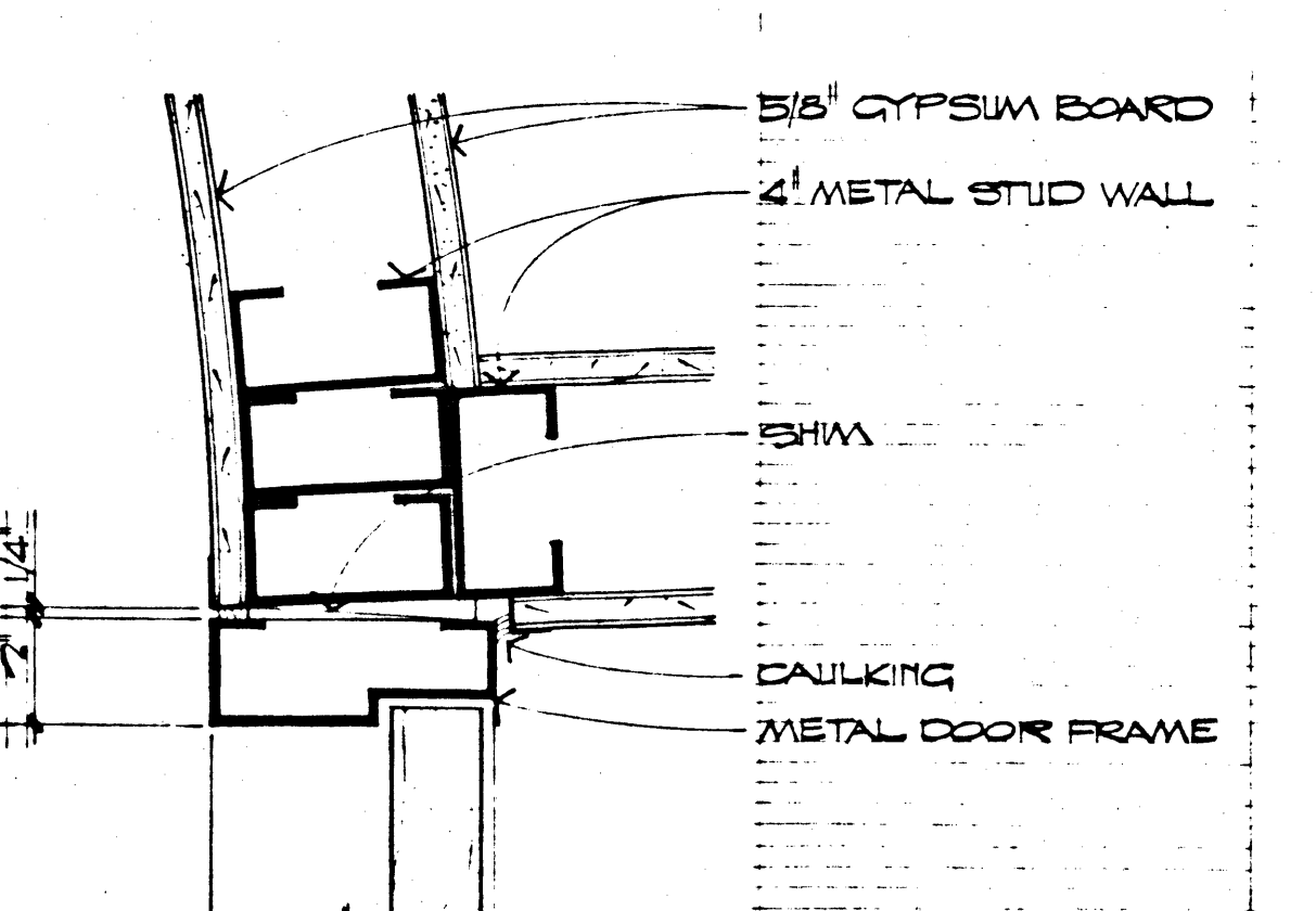
JAMB SCALE: 8" = 1'-0" 22 A-7
