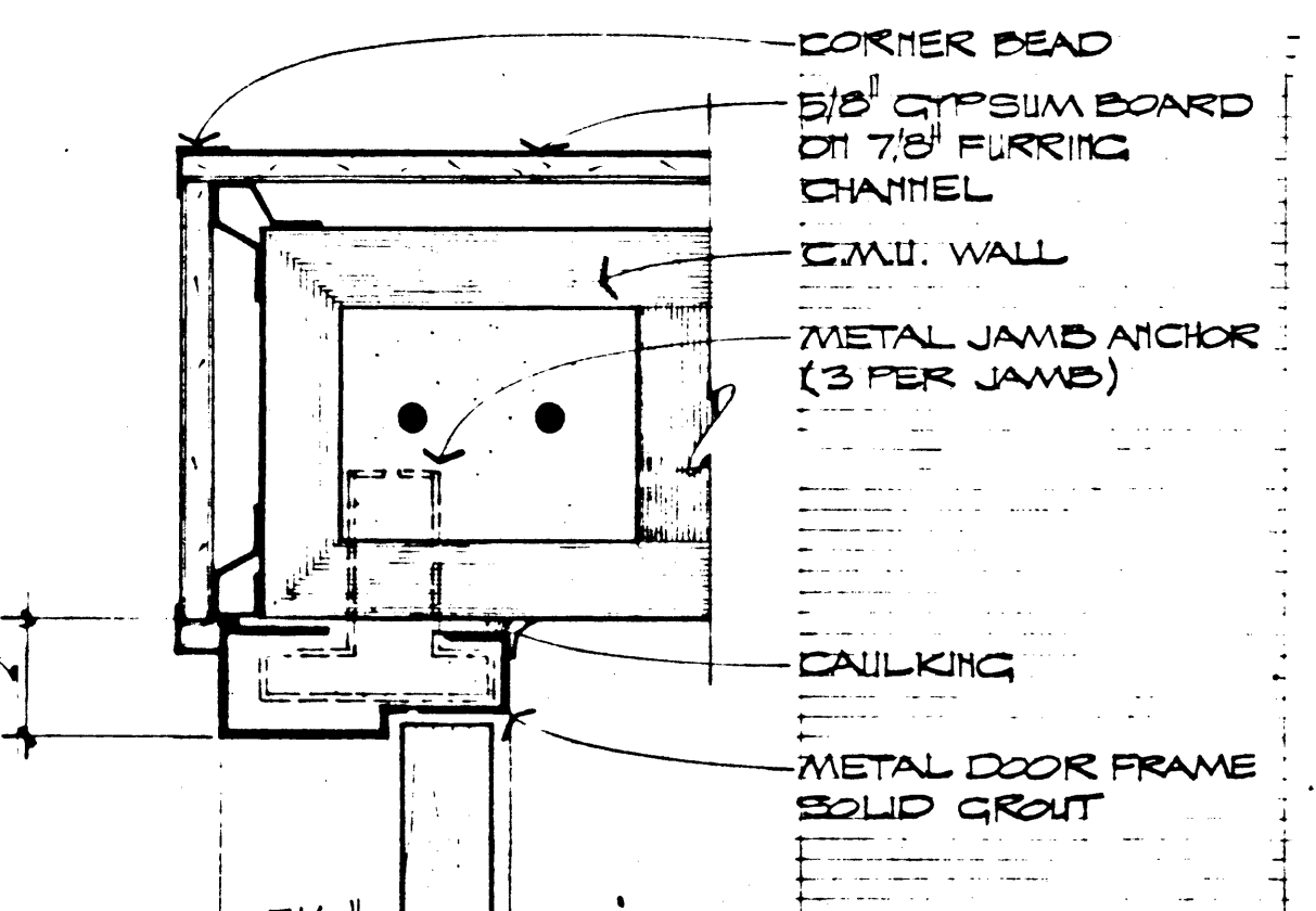
JAMB SCALE: 8" = 1'-0" 20 A-7
