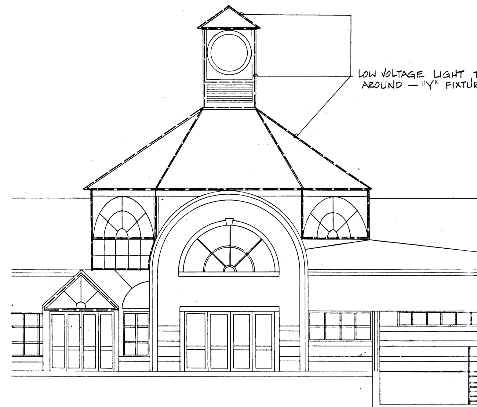
3 EAST ELEVATION SCALE: 1/8" = 1'-0" 4
