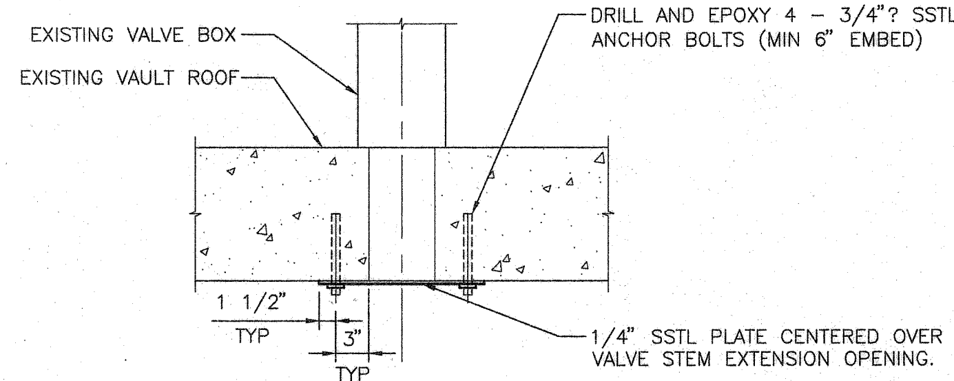
SECTION A SCALE: 1" = 1'-0"
