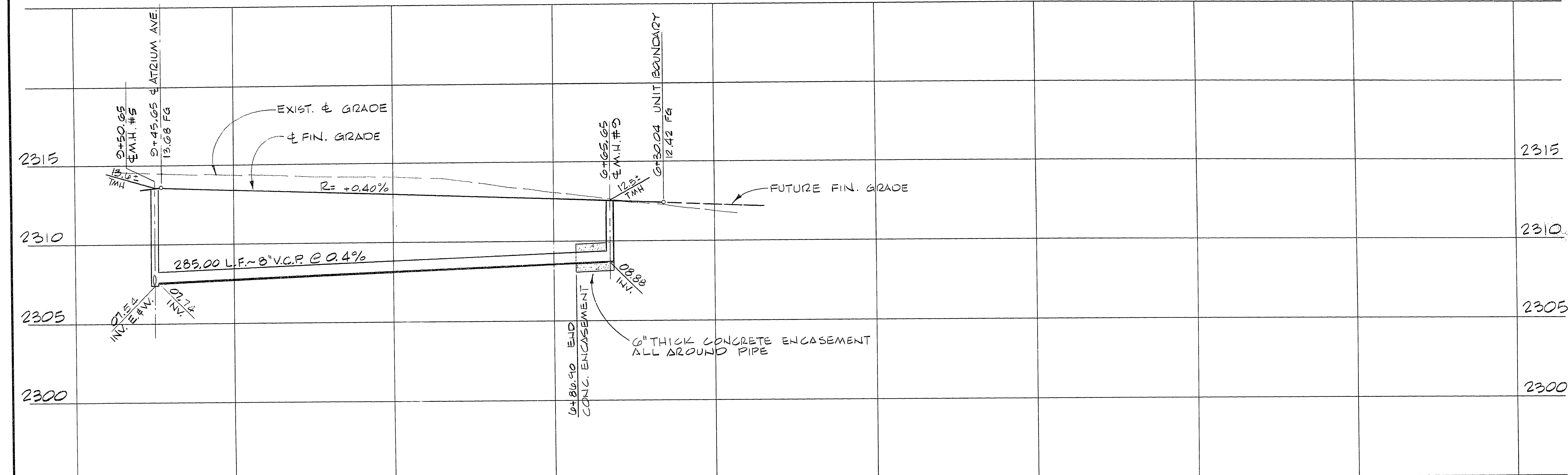
PROFILE SCALE: HORIZ. 1" = 30' VERT. 1" = 3'
