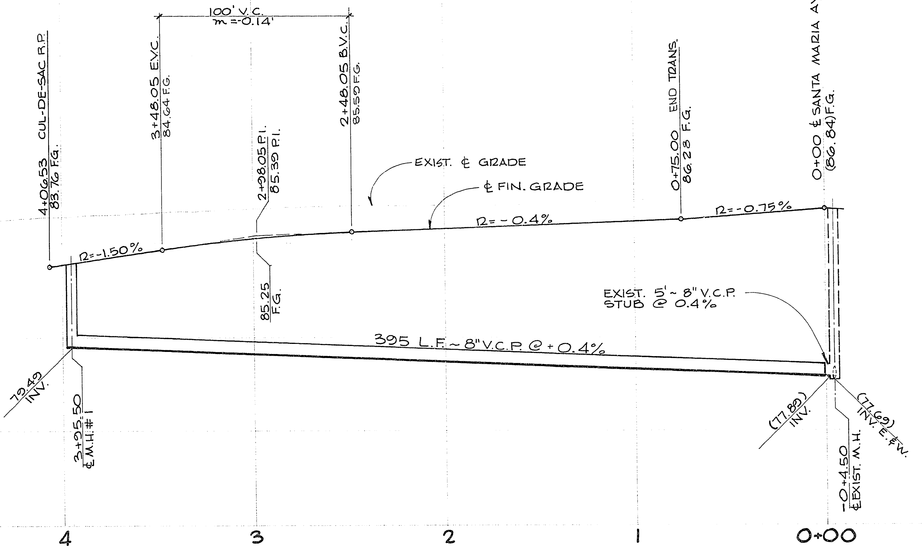
PROFILE SCALE: HORIZ.: 1"=30' VERT.: 1"=3'
