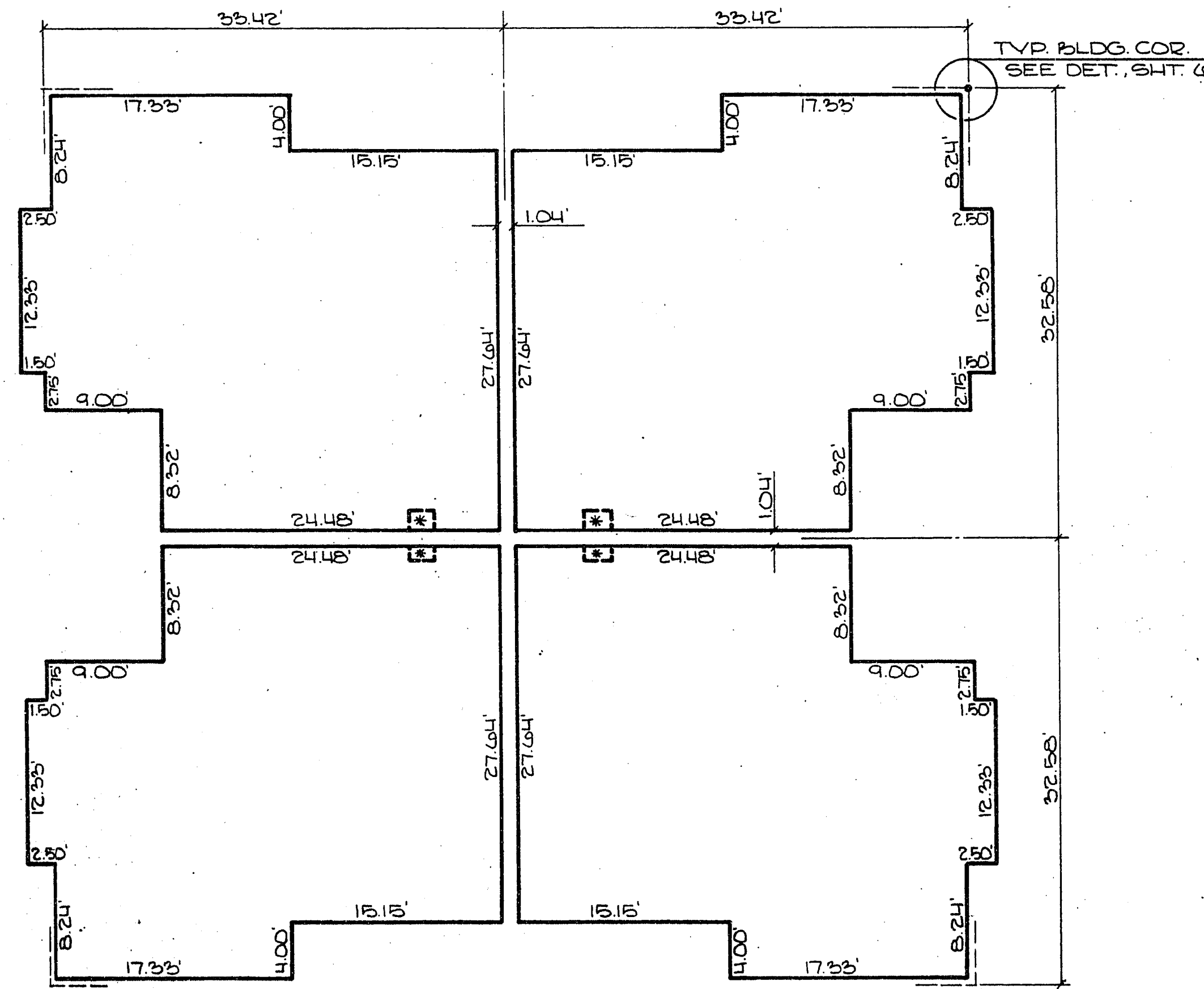
BLDG. TYPE V
