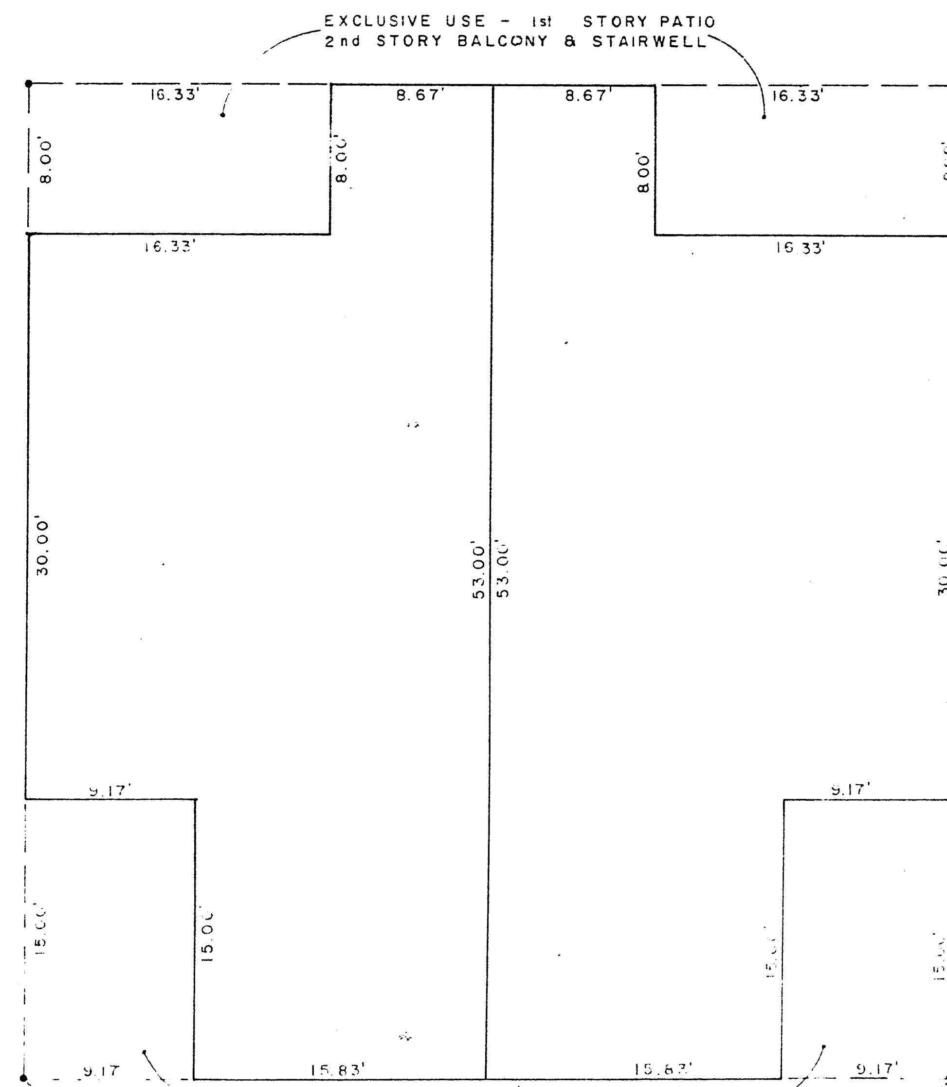
BLDG TYPE II
