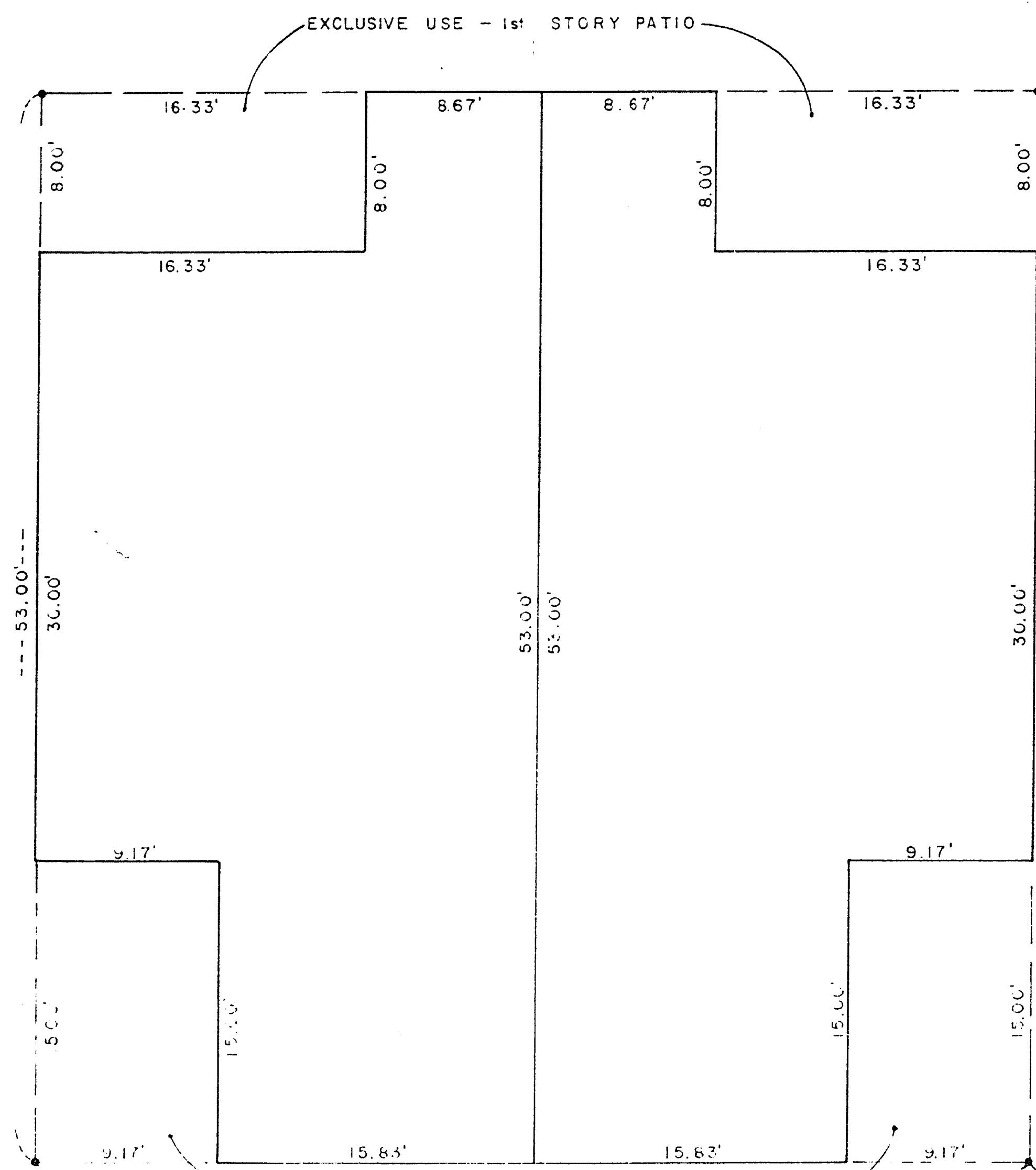
BLDG TYPE I
