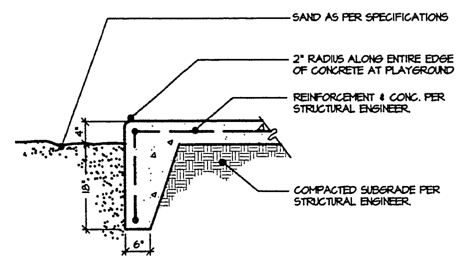
G TOT CONCRETE EDGE
