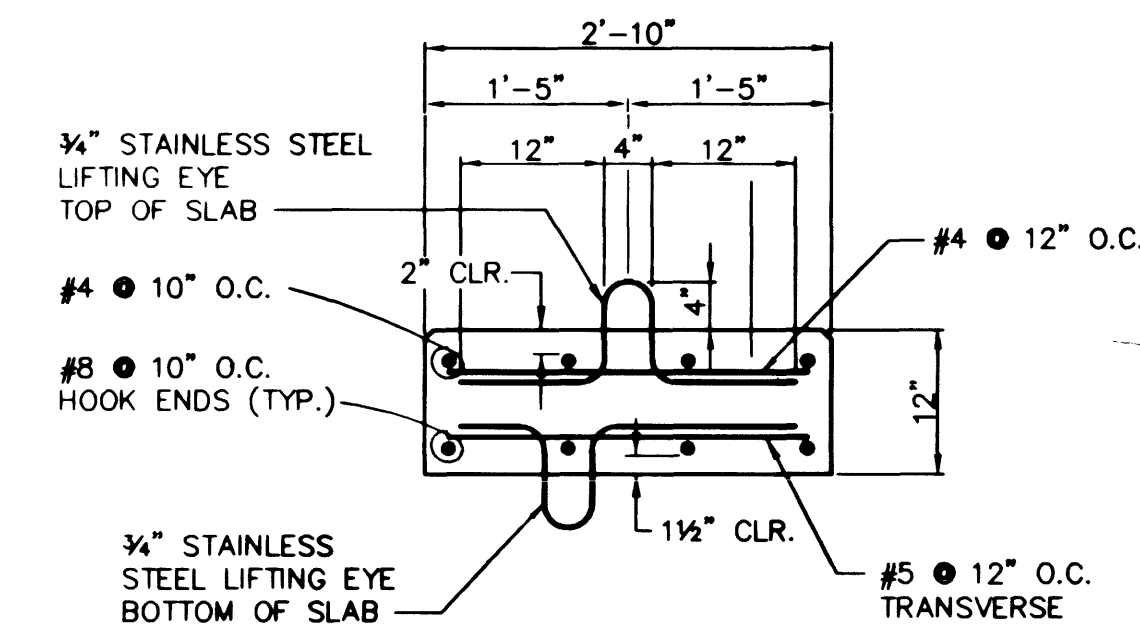
D SECTION N.T.S.
