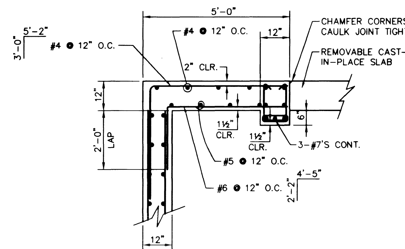
C SECTION N.T.S.
