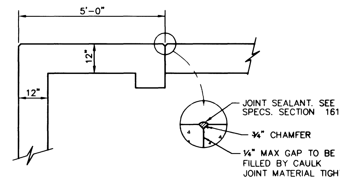
B SECTION N.T.S.
